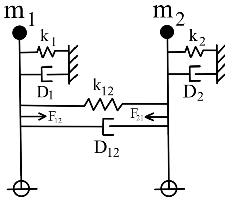
Рис. 2 математическая модель двух связанных лопаток.
