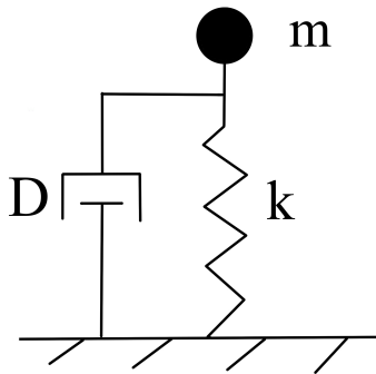
Рис. 1 схема механической системы, описывающей изолированную
