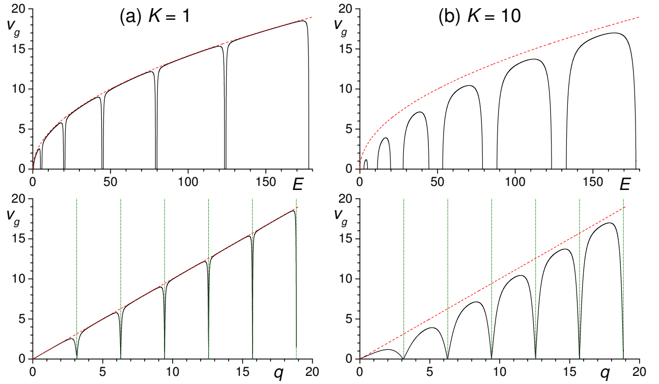
Obrázek 15: Grupová rychlost (7.4.4) v závislosti na energii (1. řádek) a na kvazihybnosti (2. řádek). Ve 2. řádku jsou hranice pásů q = \pi n znázorněny svislými zelenými čerchovanými čarami. Červená čárkovaná čára odpovídá rychlosti pro volnou částici E = \hbar q / M .
