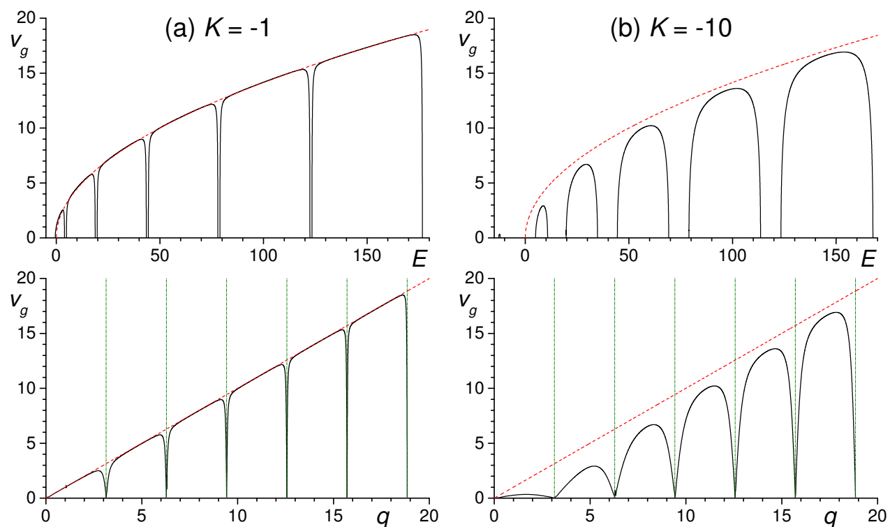
Obrázek 21: Grupová rychlost (7.4.4) v závislosti na energii (1. řádek) a na kvazihybnosti (2. řádek). Ve 2. řádku jsou hranice páسů q = \pi n znázorněny svislými zelenými čerchovanými čarami. Červená čárkovaná čára odpovídá rychlosti pro volnou částici E = \hbar q/M .
