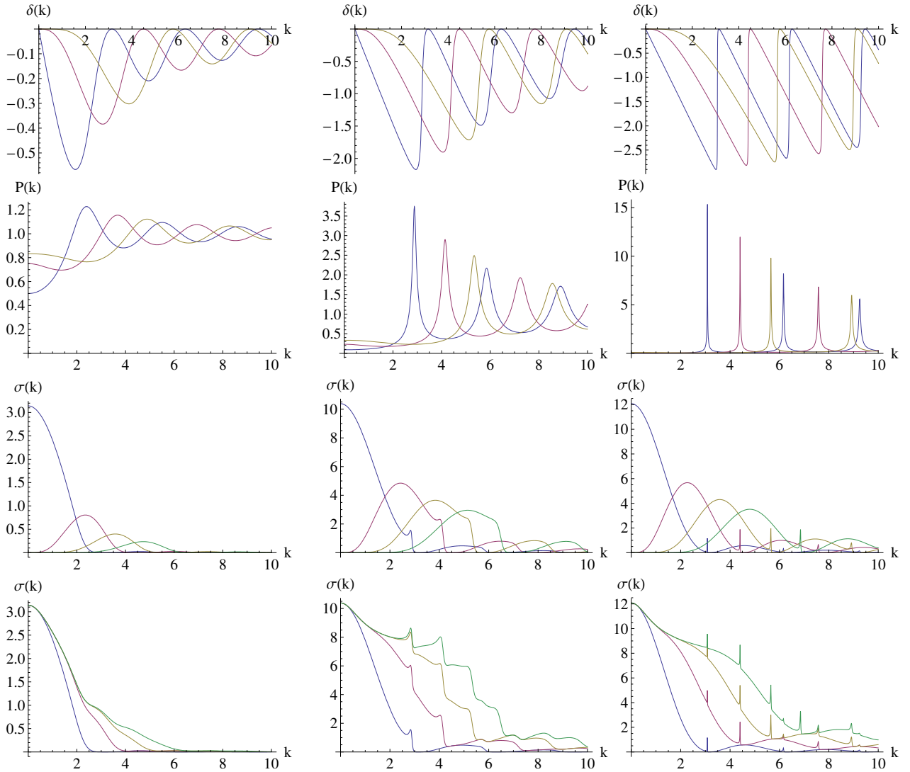
Obrázek 25: 1. řádek: Fázové posunutí l -té parciální vlny \delta_l(k) podle (13.3.14) pro l = 0 (modře), l = 1 (fialově), l = 2 (běžově). 2. řádek: Koefficient průniku l -té parciální vlny P_l(k) podle (13.3.15). 3. řádek: Účinný průřez l -té parciální vlny podle (13.3.18). 4. řádek: Součet účinných průřezů \sigma_0 (modře), \sigma_0 + \sigma_1 (fialově), \sigma_0 + \sigma_1 + \sigma_2 (běžově), \sigma_0 + \sigma_1 + \sigma_2 + \sigma_3 (zeleně). Vše je znázorněno pro různé hodnoty Q .
