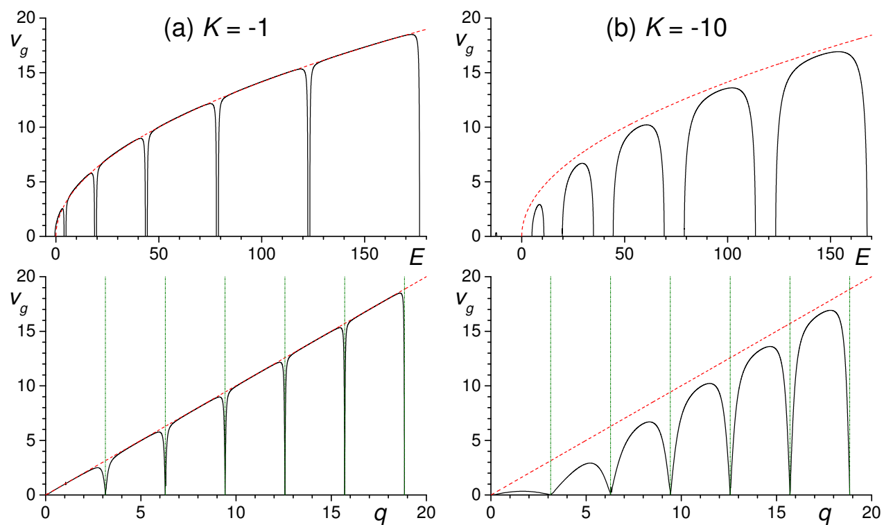
Obrázek 21: Grupová rychlost (7.4.4) v závislosti na energii (1. řádek) a na kvazihybnosti (2. řádek). Ve 2. řádku jsou hranice pásmů q = \pi n znázorněny svislými zelenými čerchovanými čarami. Červená čárkovaná čára odpovídá rychlosti pro volnou částici E = \hbar q/M .
