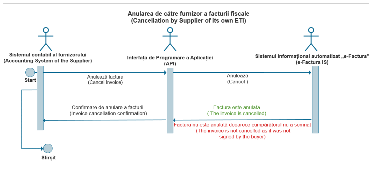
Figura 6 Procesul de anulare a facturii fiscale de către Furnizor
