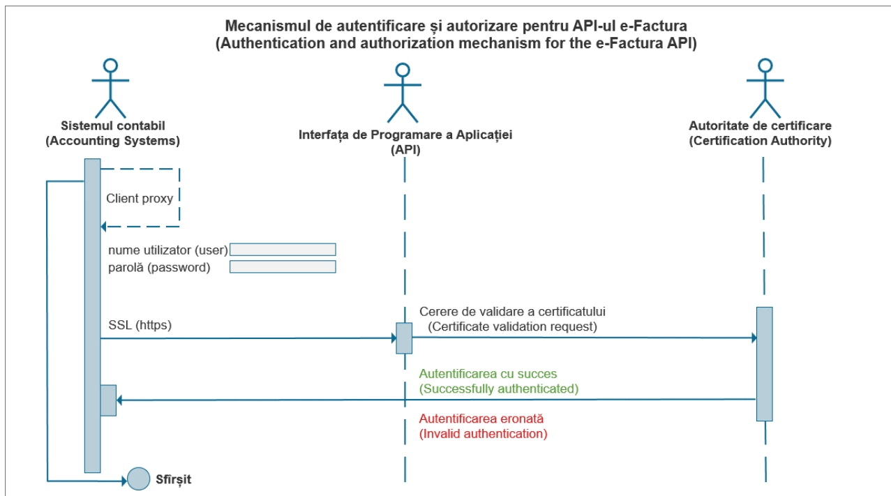
Figura 1 Mecanismul de autentificare și autorizare pentru API-ul e-Factura
