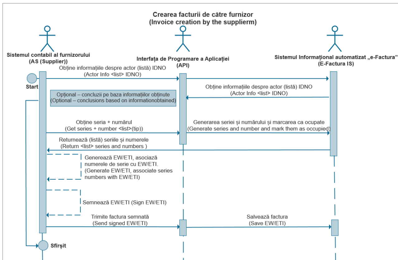
Figura 2 Crearea și semnarea facturii fiscale de către furnizor
