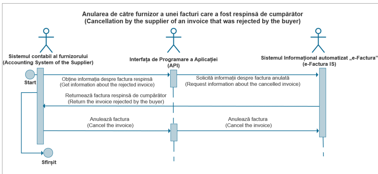
Figura 5 Anularea de către Furnizor a unei facturi fiscale respinse de către Cumpărător
