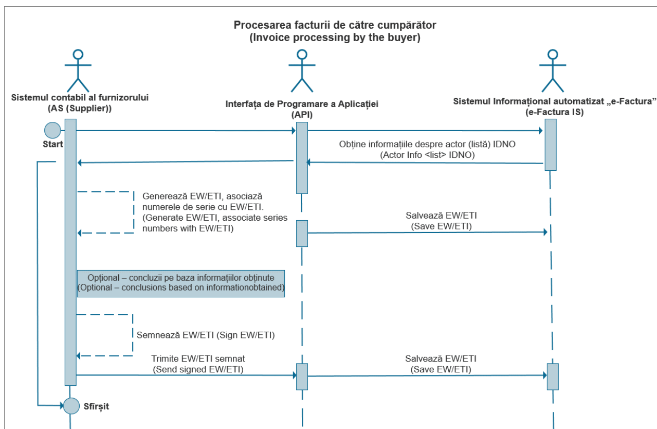
Figura 3 Procesarea facturii de către cumpărător
