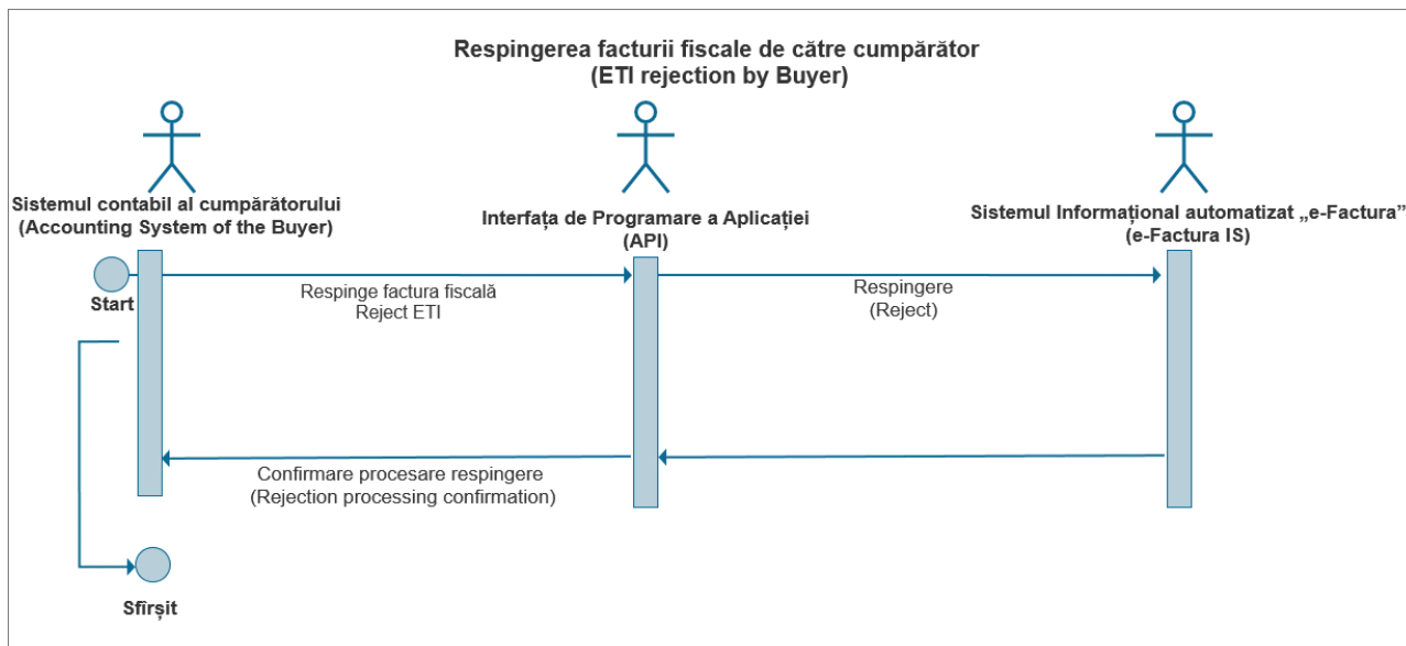
Figura 4 Respingerea facturii fiscale de către cumpărător
