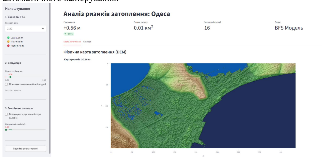
Рисунок 2.3 – сторінка карти інтерактивного веб-застосунку
