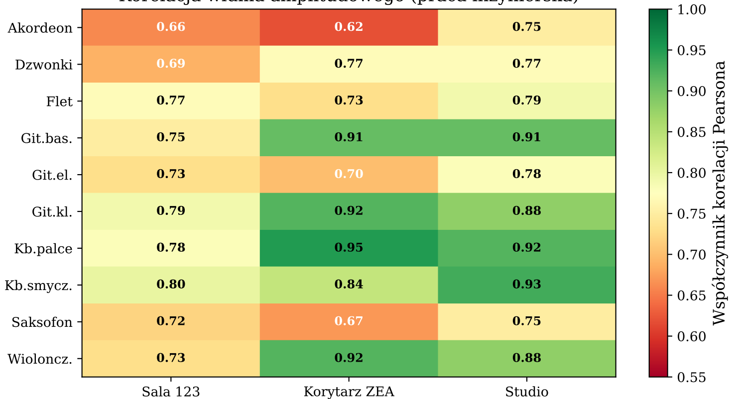
Korelacja widma amplitudowego (praca inżynierska)
