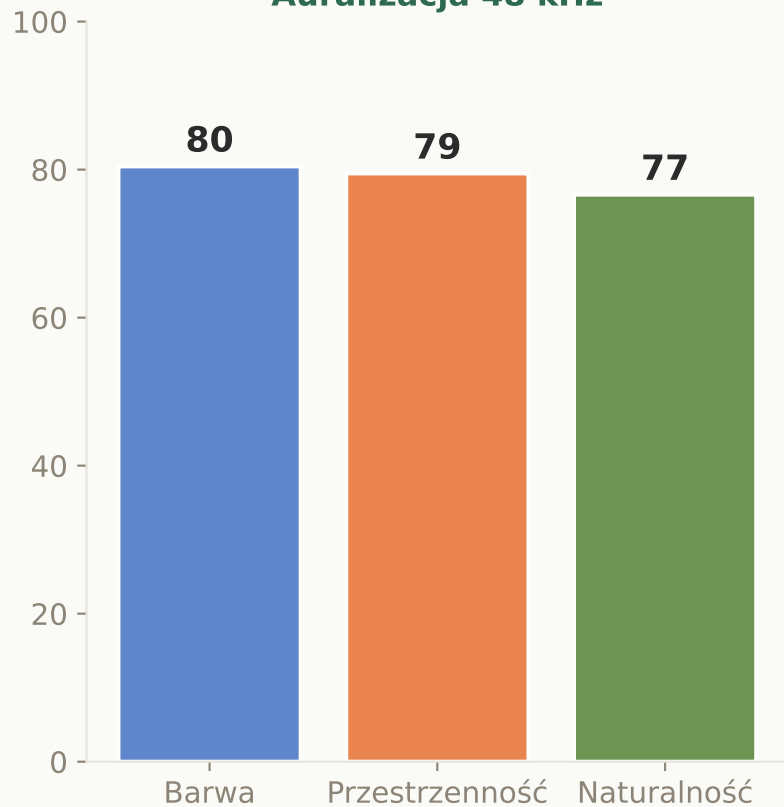
Auralizacja 48 kHz
