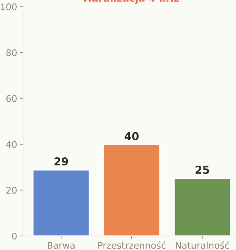
Auralizacja 4 kHz
