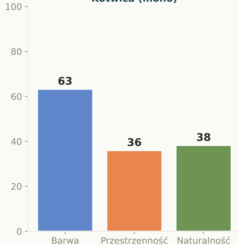
Kotwica (mono)
