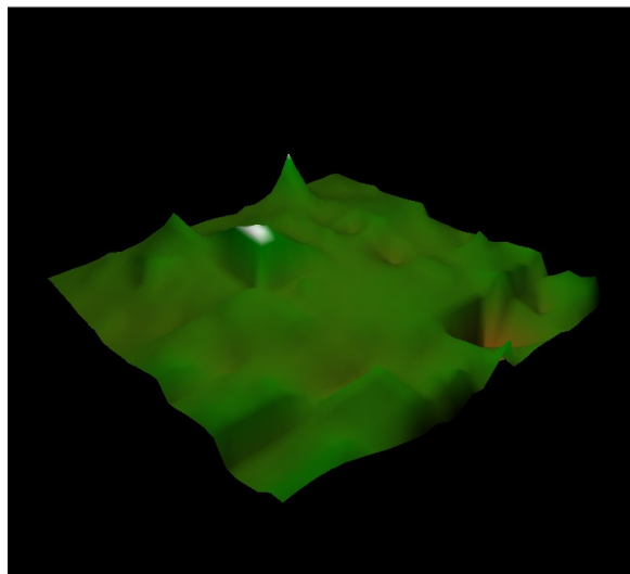
0 итераций
