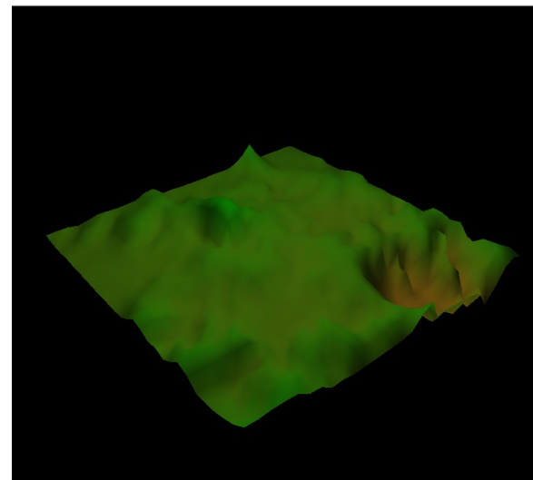
100 итераций
