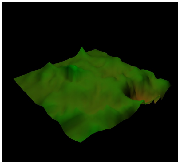
50 итераций
