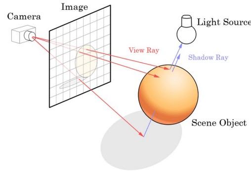
Трассировка лучей
