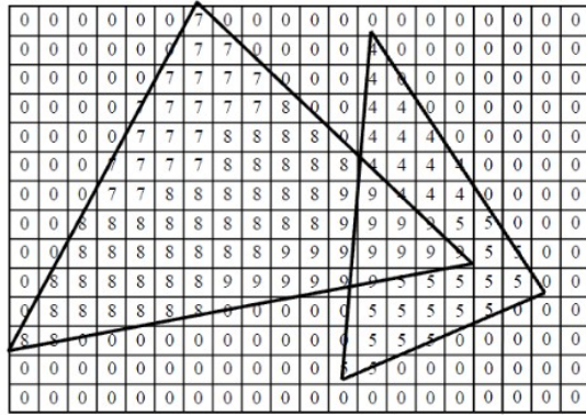
Z-буфер
