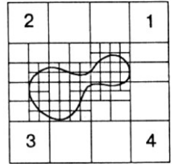
Алгоритм Варнока
