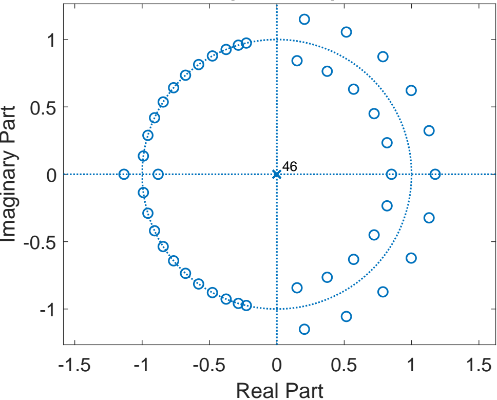
FIR pole-zero plot
