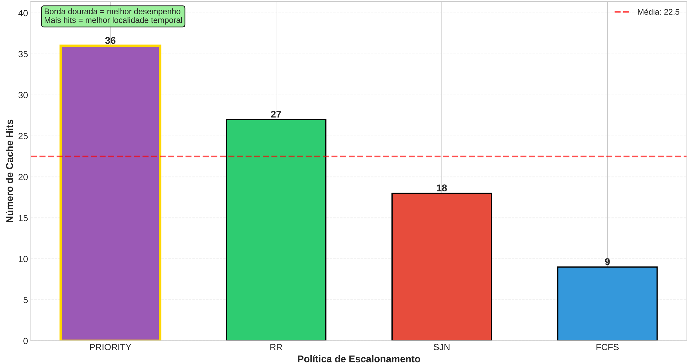
Cache Hits por Escalonador (maior é melhor - dados encontrados na cache)
