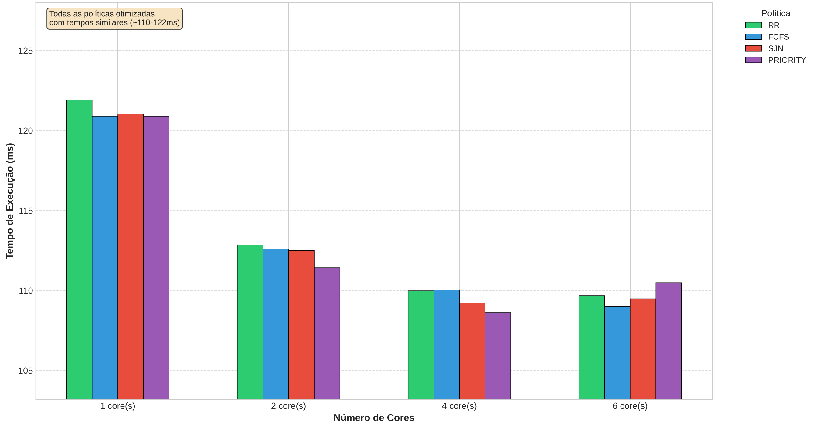
Comparativo de Tempo de Execução: 4 Políticas × 4 Configurações de Cores (menor é melhor)
