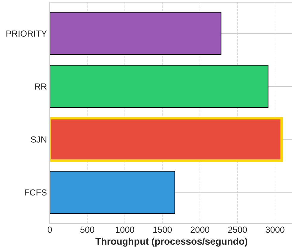
Throughput (maior é melhor)
