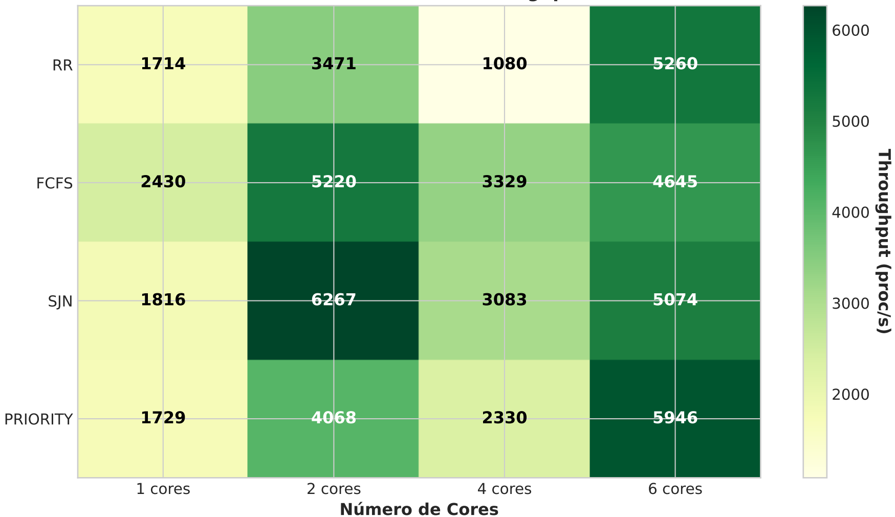
Heatmap: Throughput por Política e Cores (verde escuro = maior throughput)
