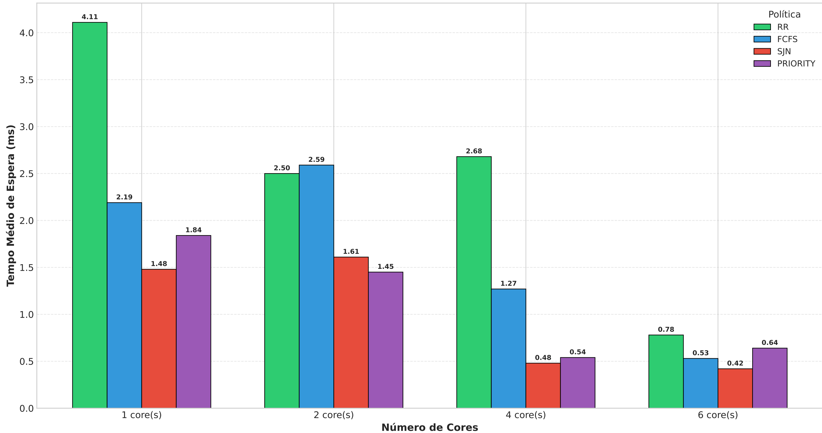
Tempo Médio de Espera por Política e Número de Cores
