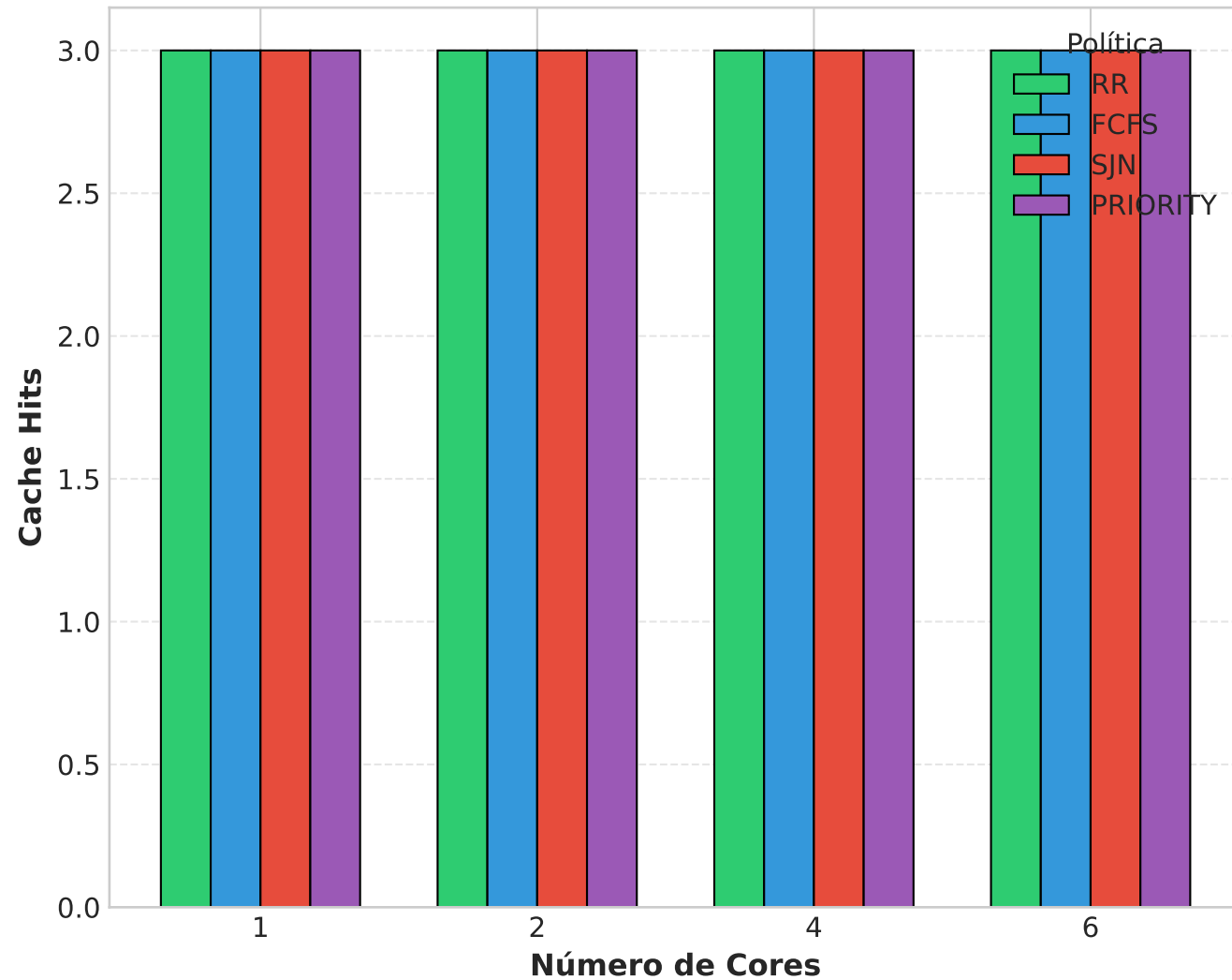
Cache Hits por Política e Cores
