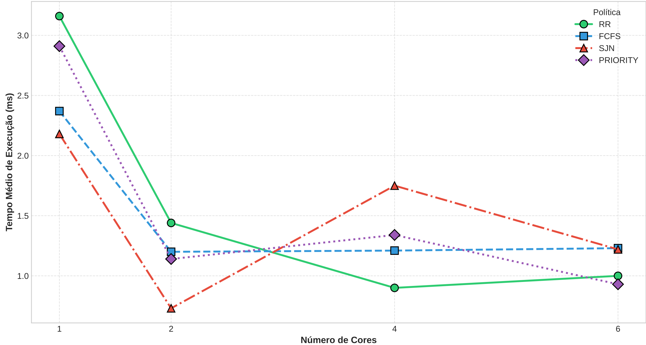
Tempo Médio de Execução vs Número de Cores (menor é melhor)
