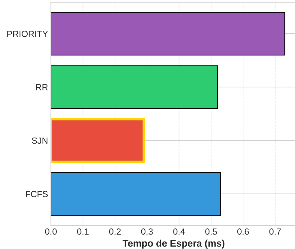
Tempo Médio de Espera (menor é melhor)
