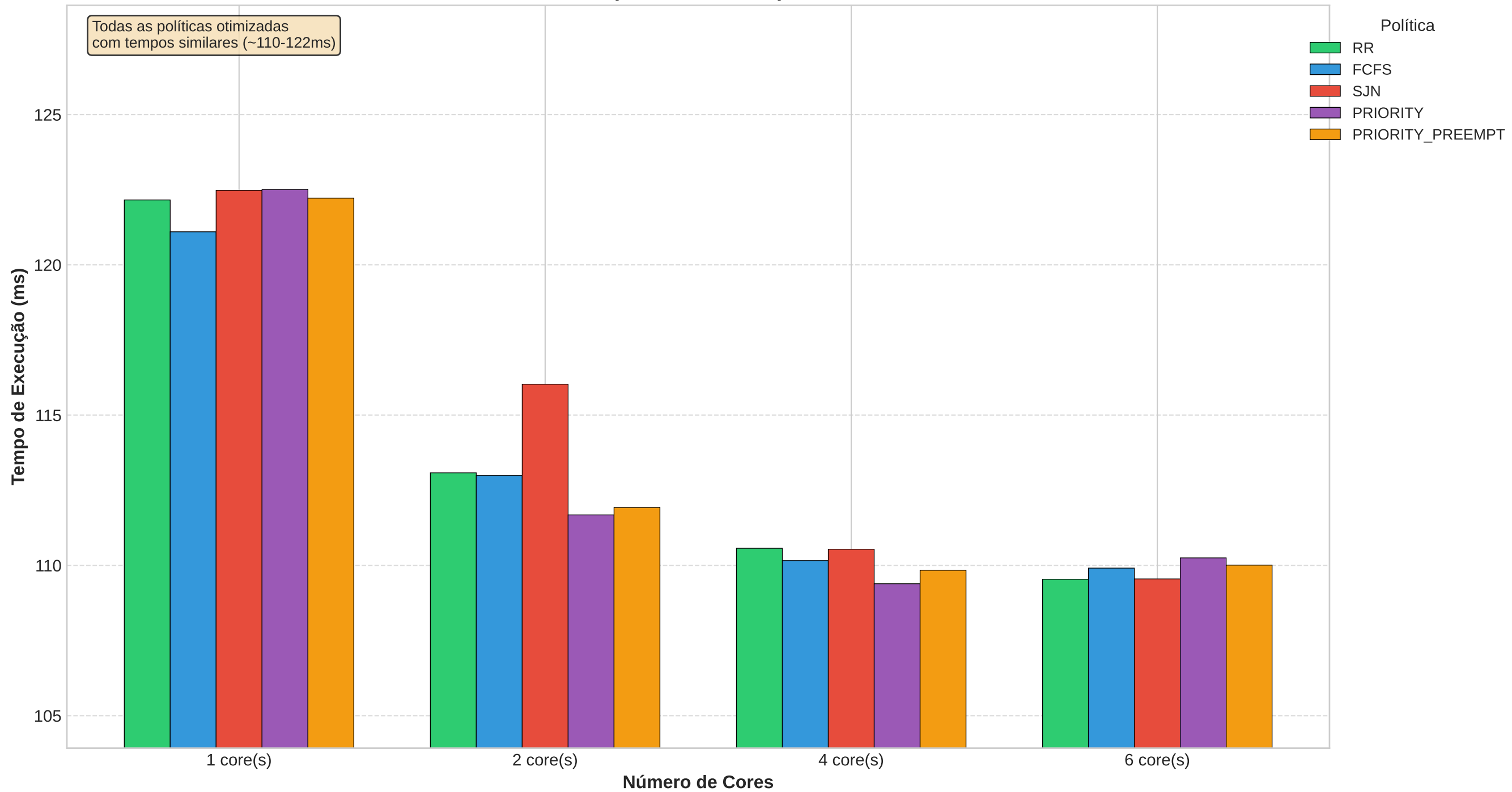
Comparativo de Tempo de Execução: 5 Políticas × 4 Configurações de Cores (menor é melhor)
