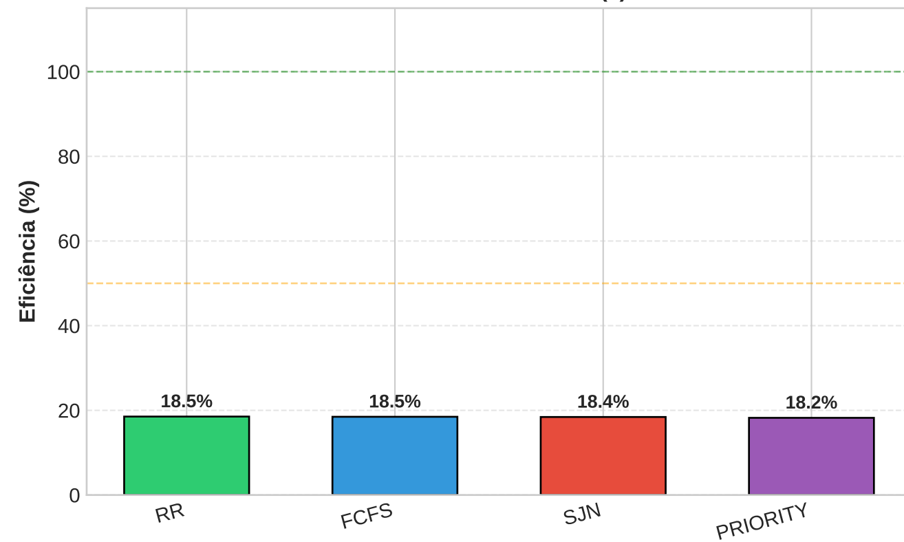
Eficiência com 6 Core(s)
