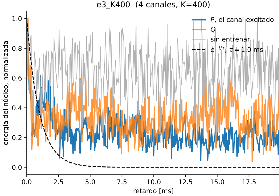
Figura 1: Energía del núcleo FIR aprendido en función del retardo, sobre act1 , corrida e3_K400 (cuatro canales, K = 400 muestras, 20 ms). La energía es la norma sobre los cuatro canales para cada retardo, normalizada a su máximo; los canales por separado no son comparables porque la red que sigue puede reescalar cualquiera de ellos sin cambiar la función. La curva gris es el mismo filtro sin entrenar, y sirve de control para distinguir estructura de ruido. La curva negra punteada es la respuesta al impulso del actuador verdadero, e^{-t/\tau} con \tau = 1,0 ms, que el entrenamiento nunca vio.
