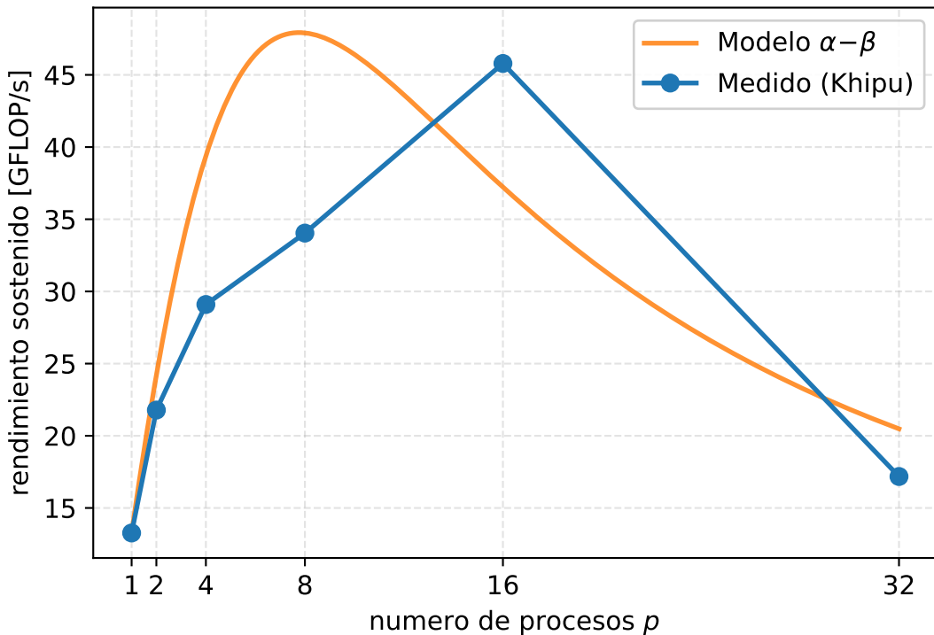
FLOP/s vs procesos (region paralelizable)
