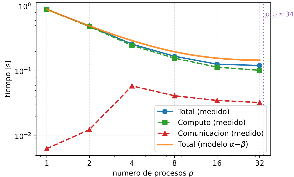
Tiempo de ejecucion vs procesos (n=14376, k=7)
