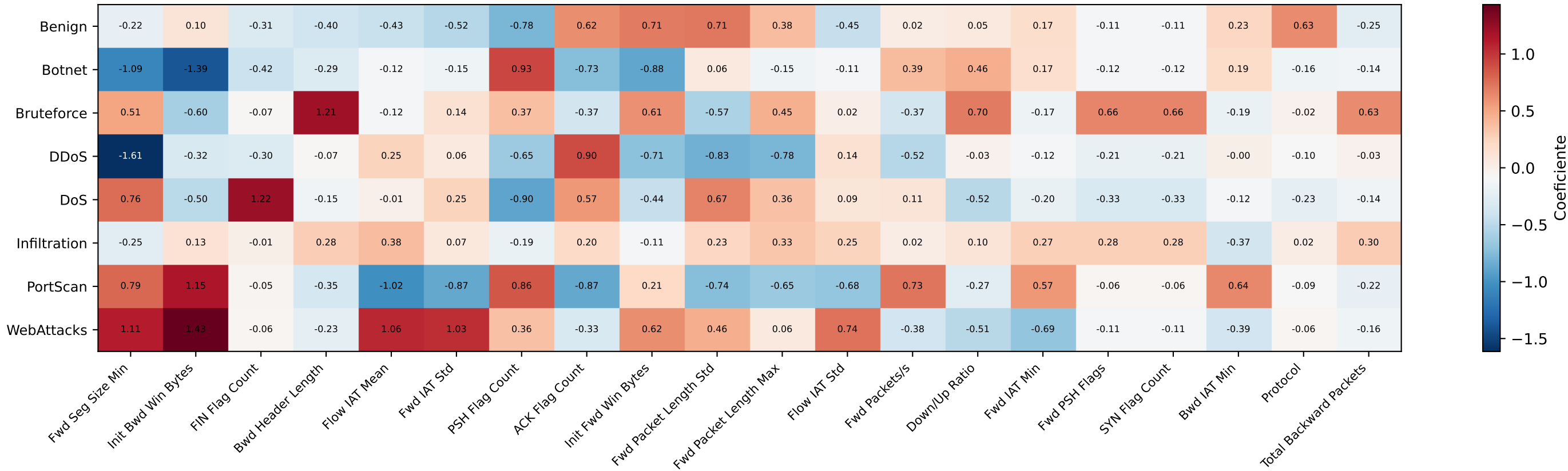
Heatmap de Coeficientes — Top 20 Features × Classes (Azul = contribui para BENIGNO | Vermelho = contribui para ATAQUE)
