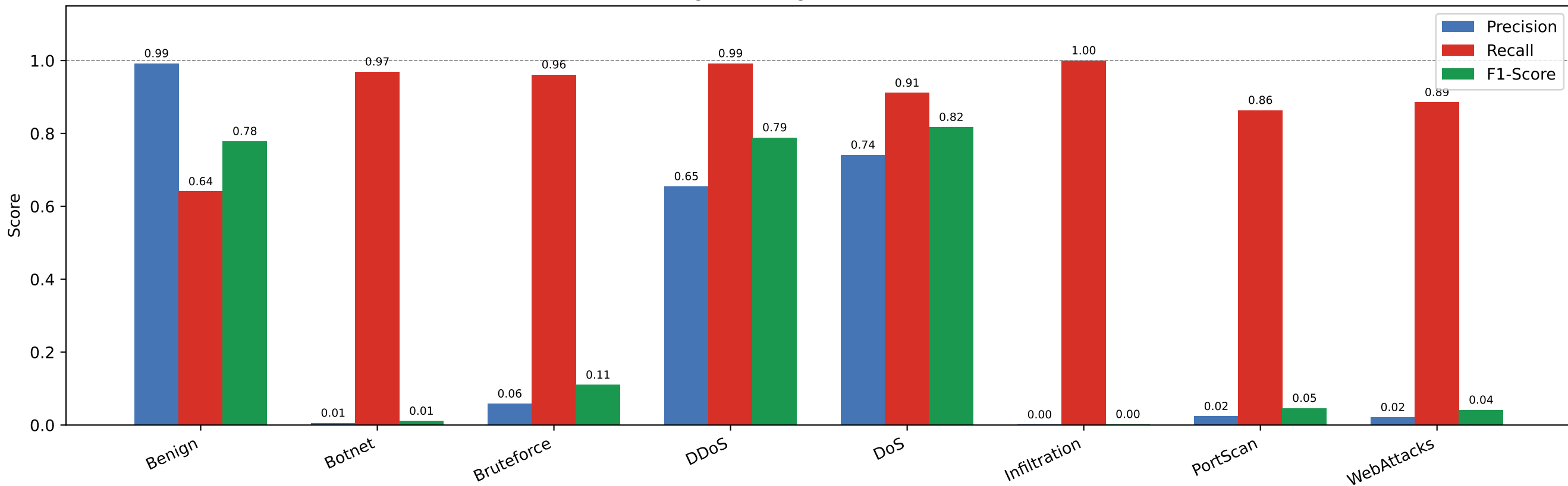
Precision, Recall e F1-Score por Classe (Regressão Logística Multiclasse)
