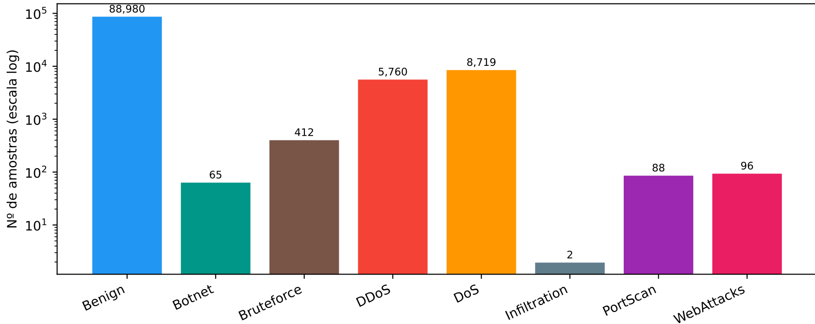
Distribuição de Amostras no Conjunto de Teste por Classe
