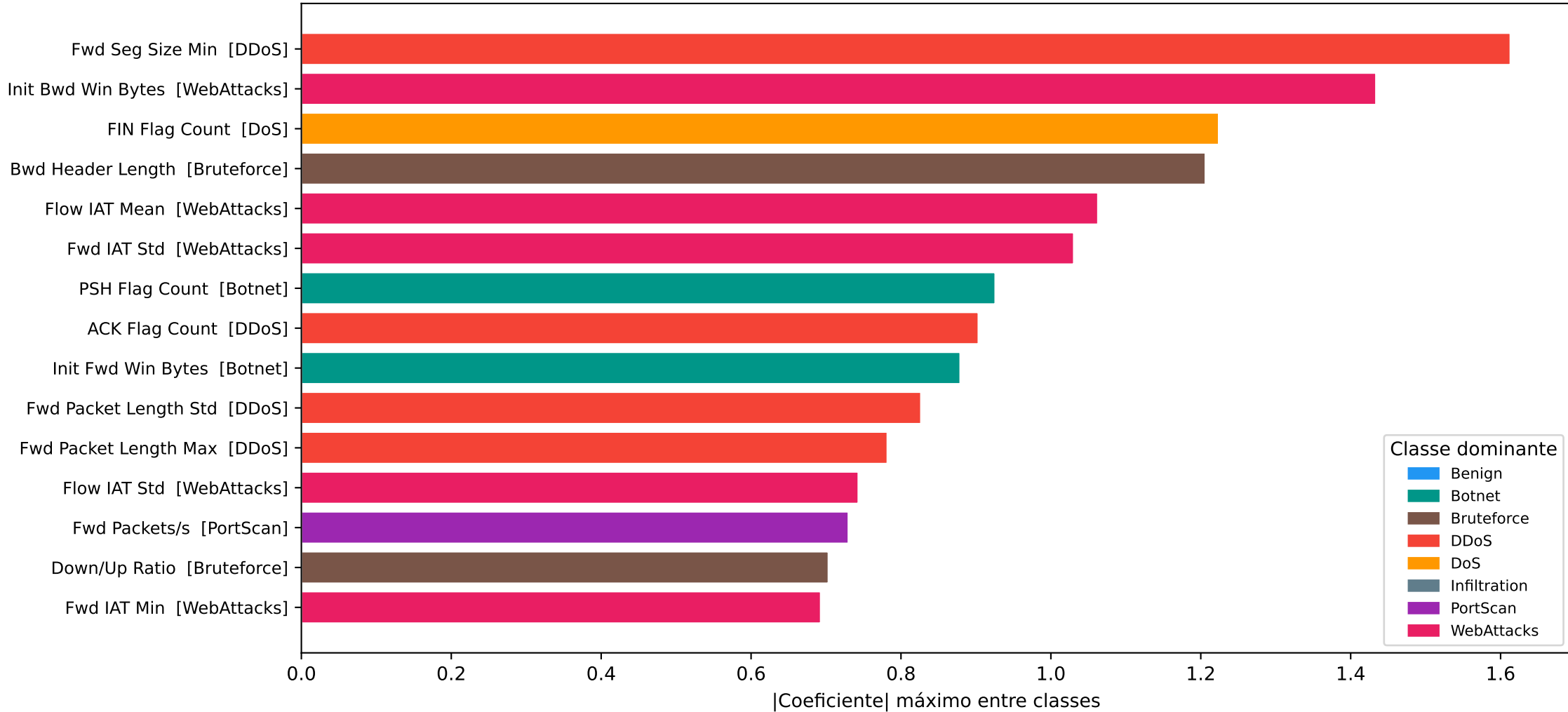
Top 15 Features — Importância Global (Cor indica a classe que mais discrimina)
