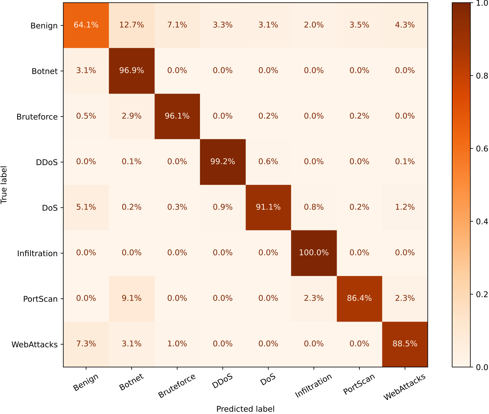
Matriz de Confusão — Normalizada por Linha (Taxa de Acerto por Classe Real)
