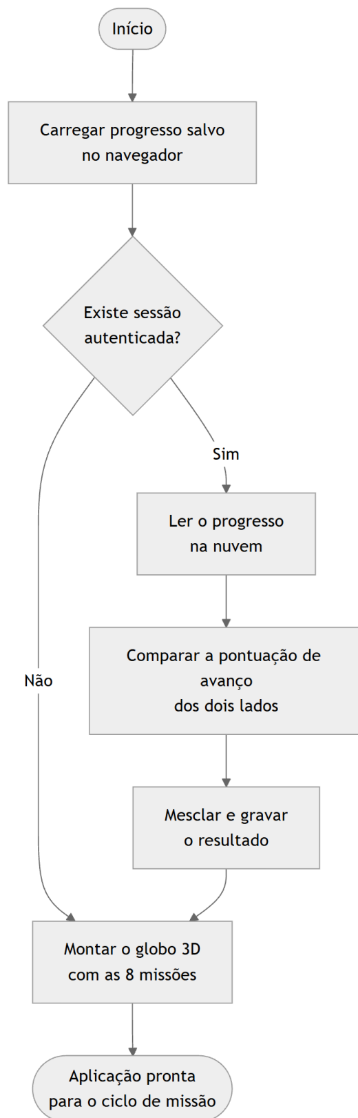
Figura 1 - Fluxograma de inicialização da aplicação
