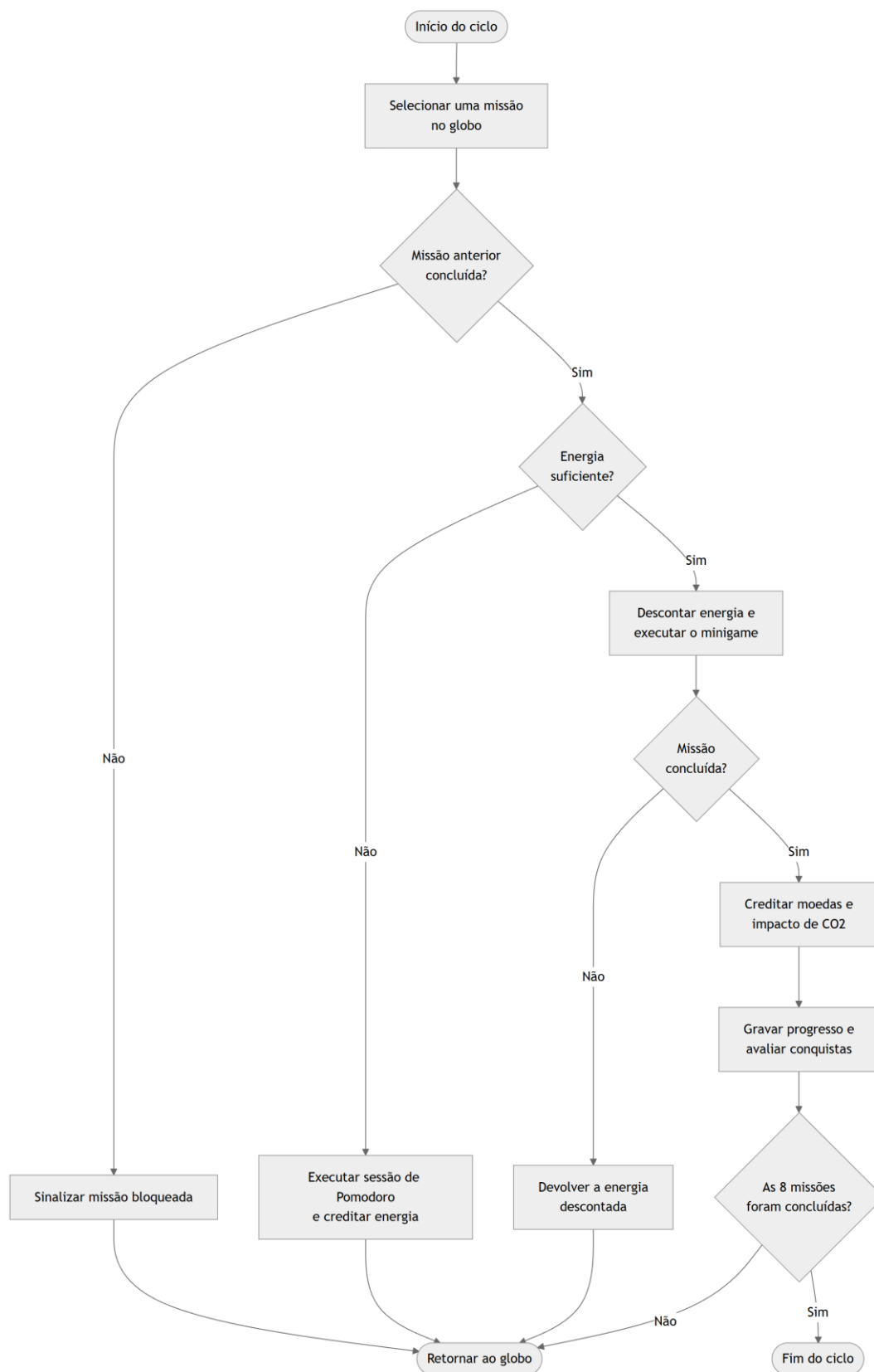
Figura 2 - Fluxograma do ciclo de missão
