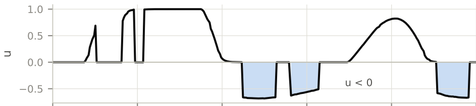
PWM reconstruído
