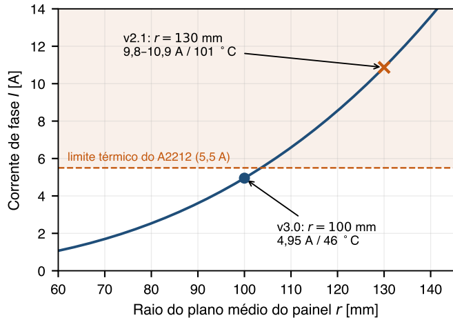
(b) custo do raio a 1800 rpm ( I \propto r^3 )
