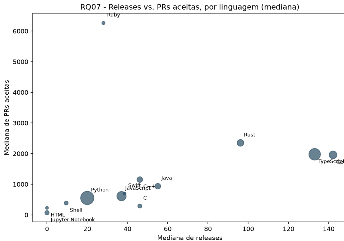
Figura 7 — Releases e PRs aceitas por linguagem (RQ07).
