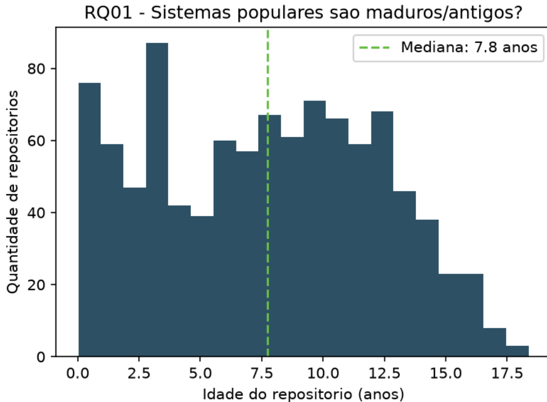
Figura 1 — Distribuição da idade dos repositórios (RQ01).
