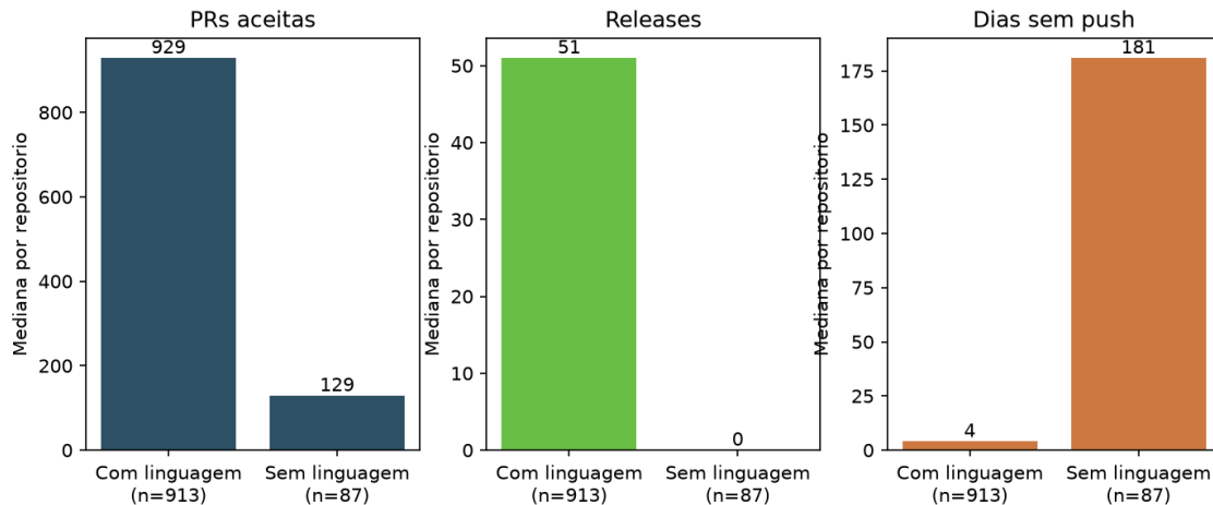
Figura 9 — Indicadores de manutenção por presença de linguagem primária (RQ08).
