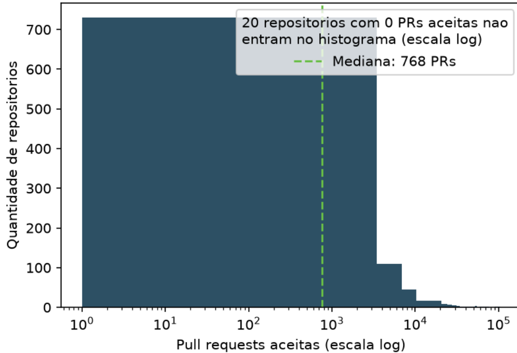
Figura 2 — Distribuição de Pull Requests aceitas (RQ02).
