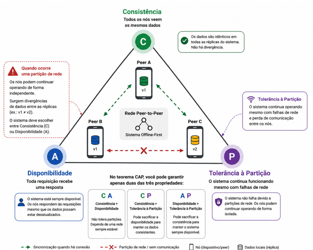
Figura 3: MODELO CAP NA VISÃO DE SISTEMAS OFFLINE-FIRST
