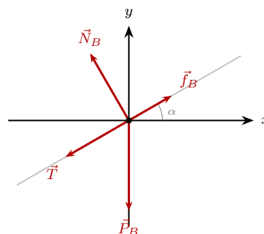
fuerzas sobre B
