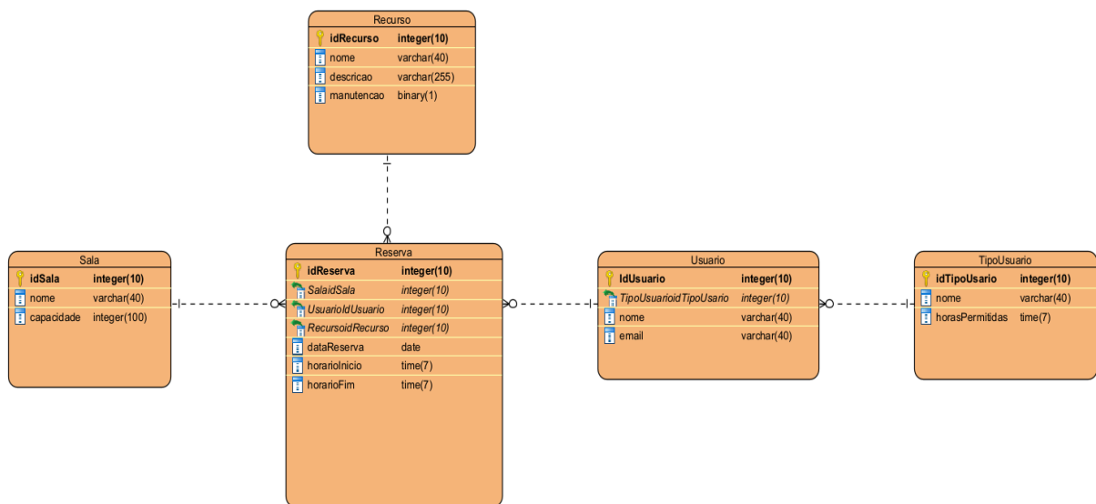
Diagrama Banco de dados SQL Server:
