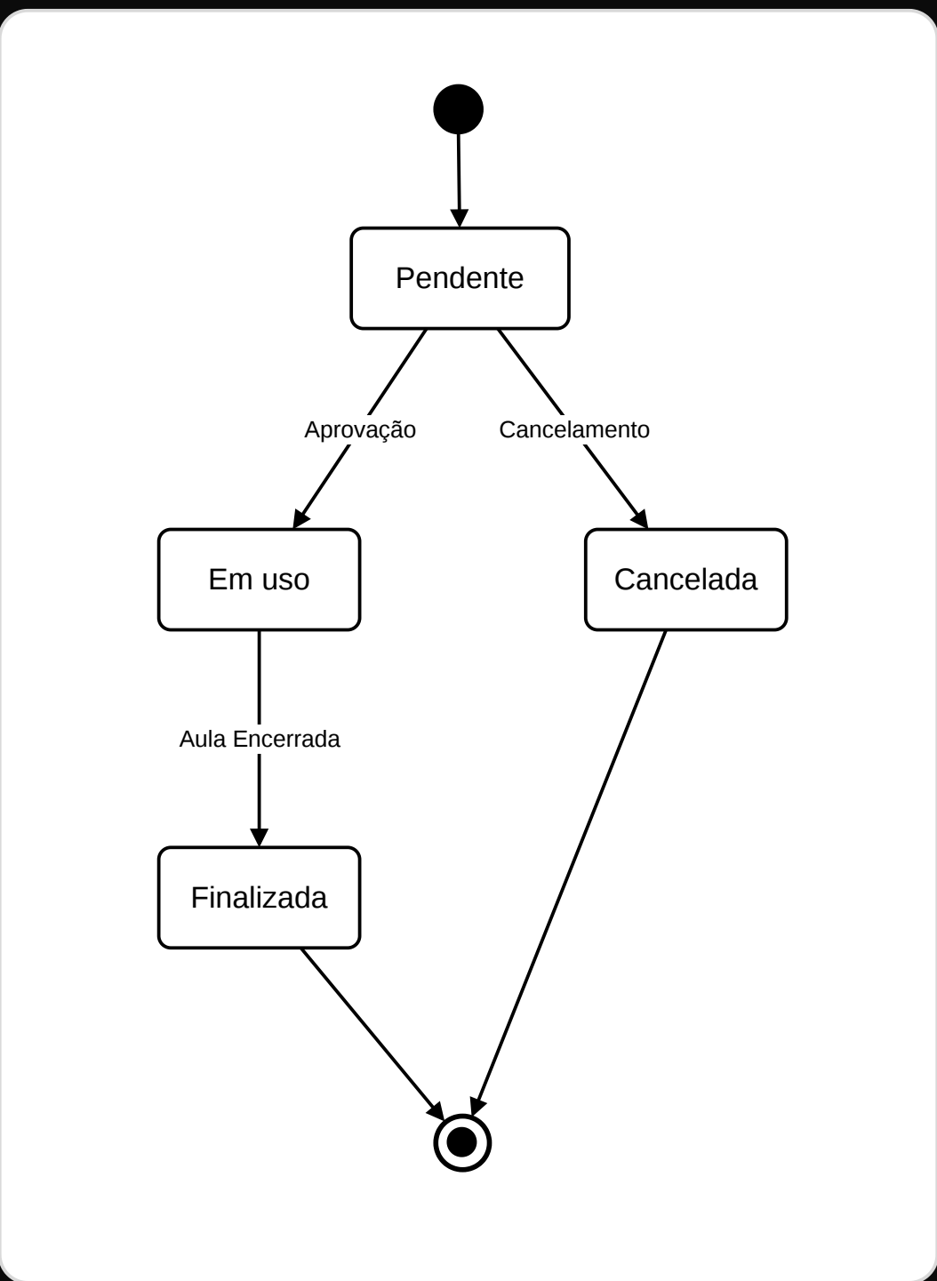
Diagrama de Estado
