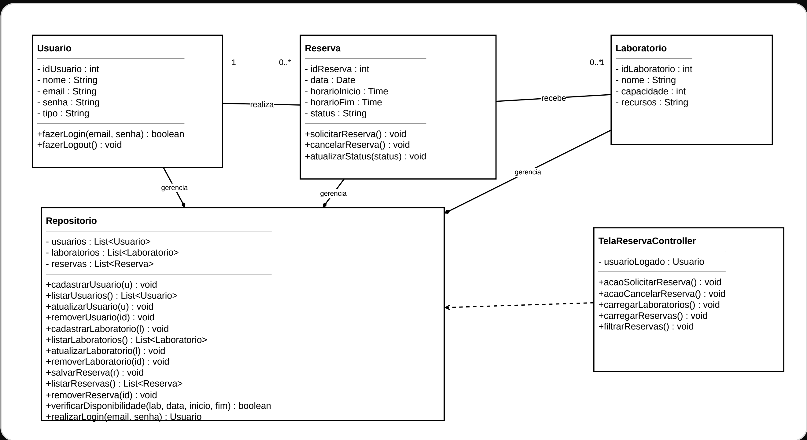
Diagrama De Classe
