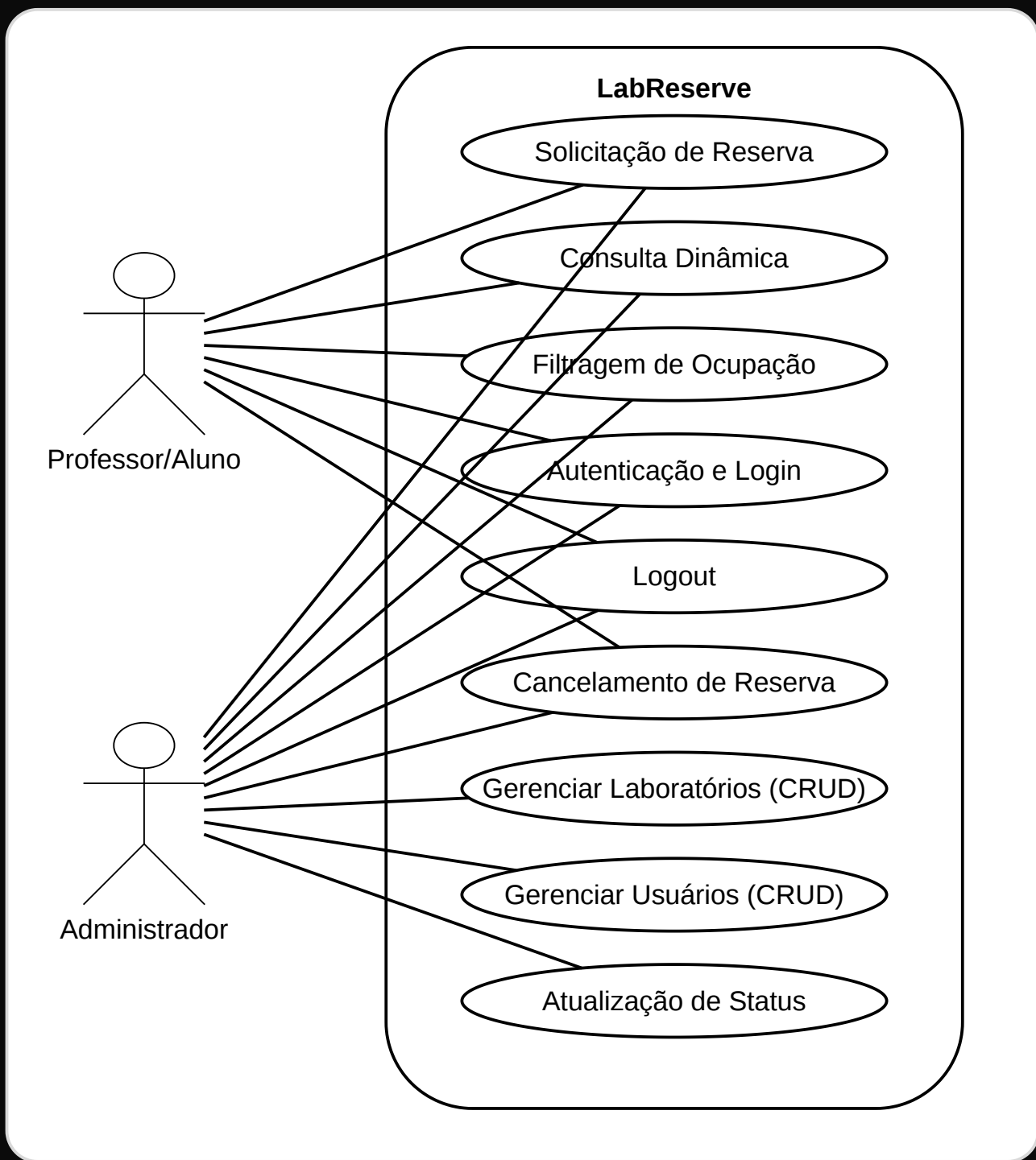
Diagrama Casos de Uso
