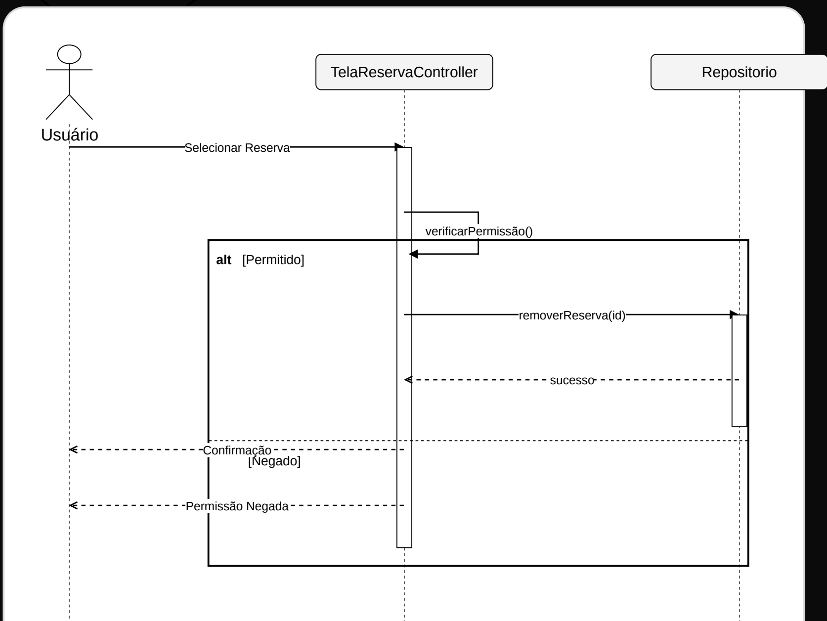
Diagrama de Sequencia Cancela Reserva
