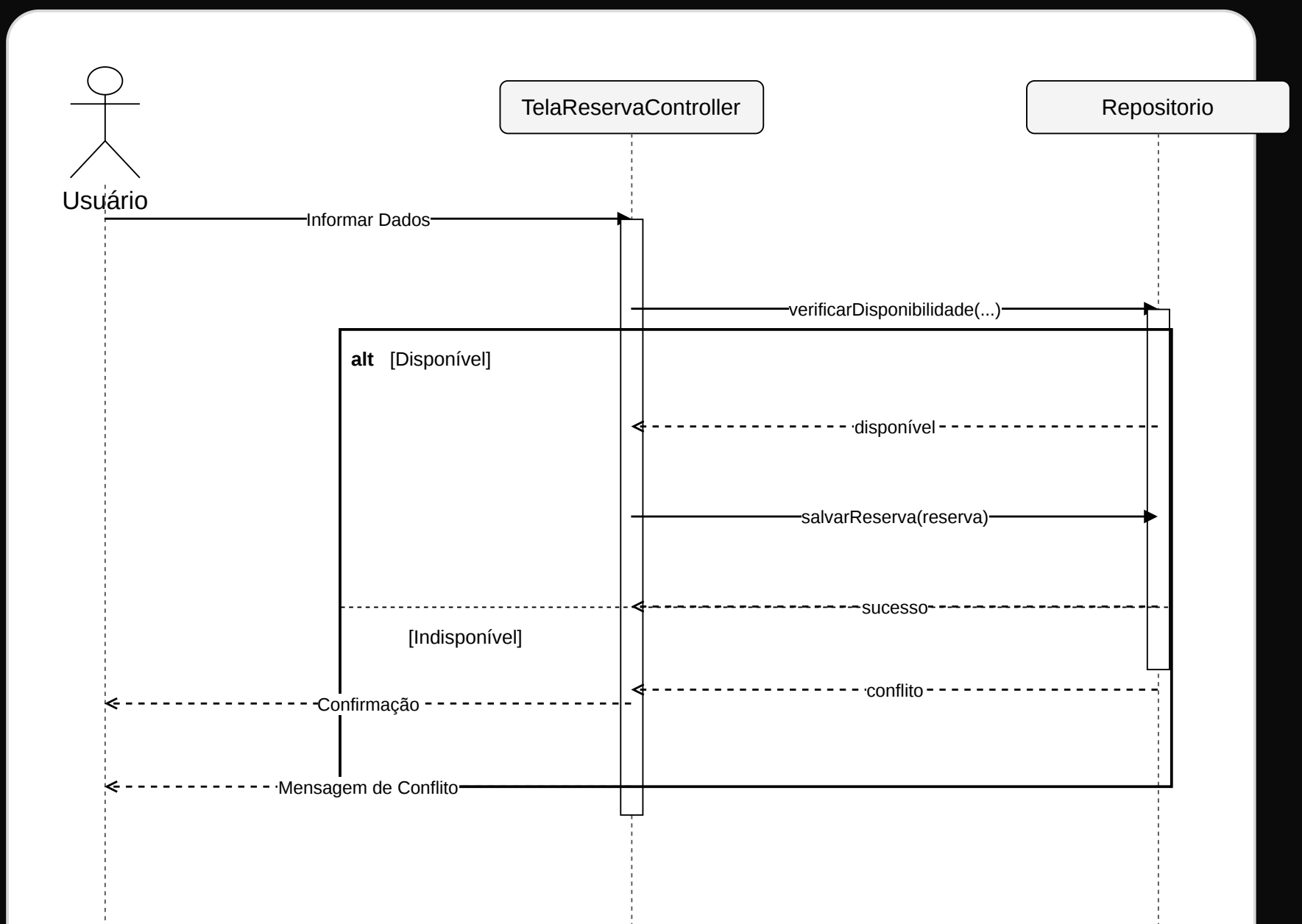
Diagrama de Sequencia Solicita Reserva
