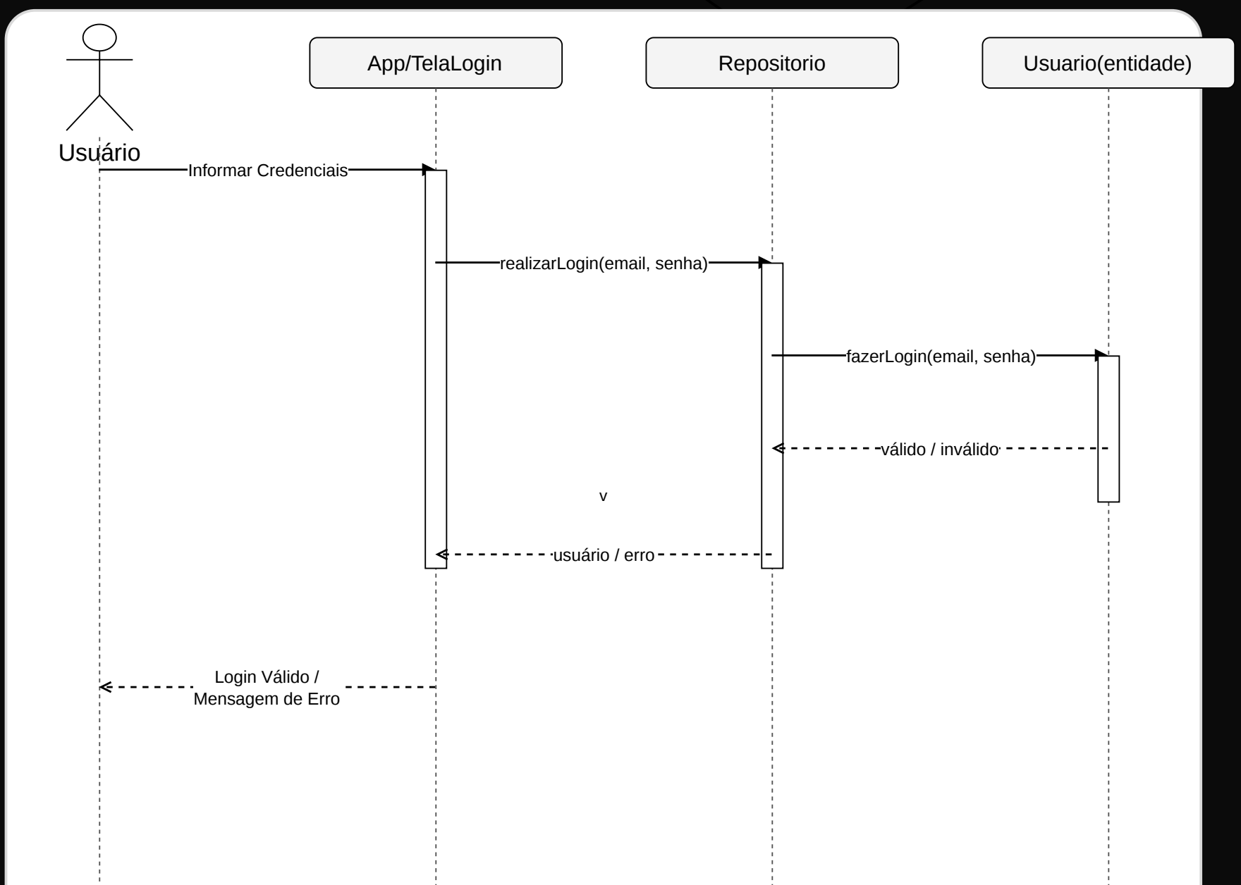
Diagrama de Sequencia Login
