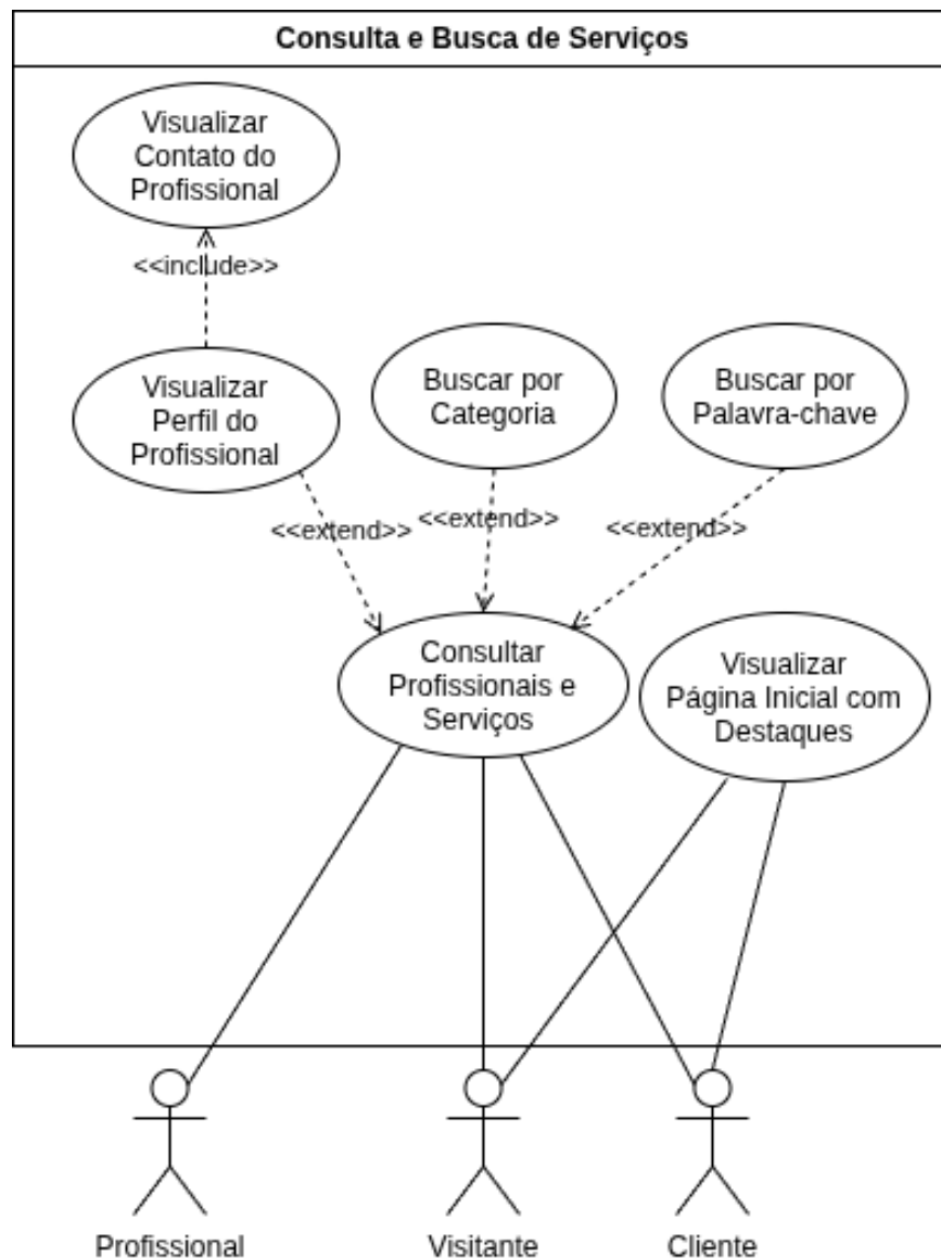
Figura 3 — Diagrama de casos de uso do módulo Consulta e Busca de Serviços
