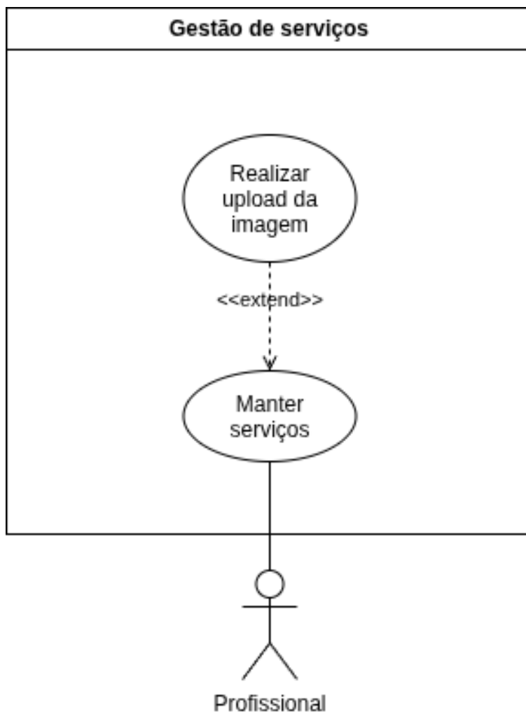
Figura 2 — Diagrama de casos de uso do módulo Gestão de Serviços
