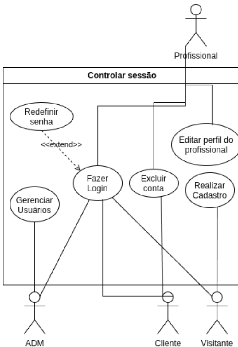
Figura 1 — Diagrama de casos de uso do módulo Gestão de Usuários
