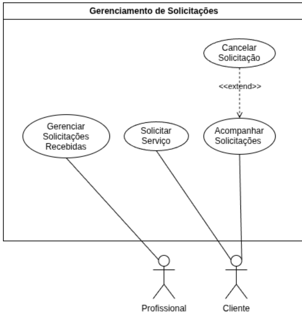
Figura 6 — Diagrama de casos de uso do módulo Gerenciamento de Solicitações
