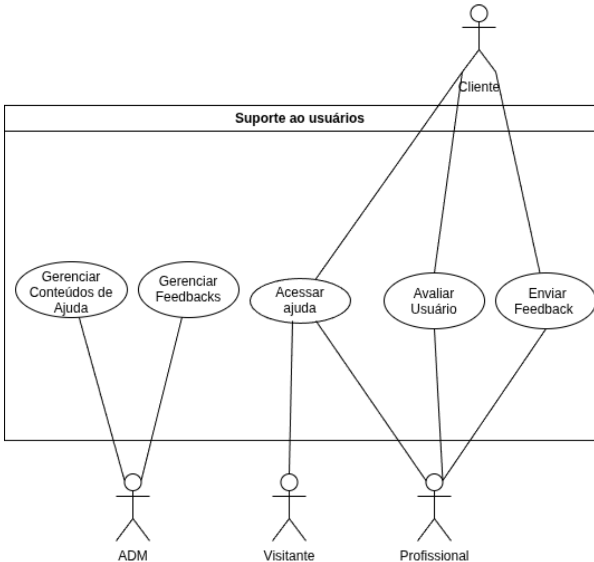
Figura 5 — Diagrama de casos de uso do módulo Suporte ao Usuário
