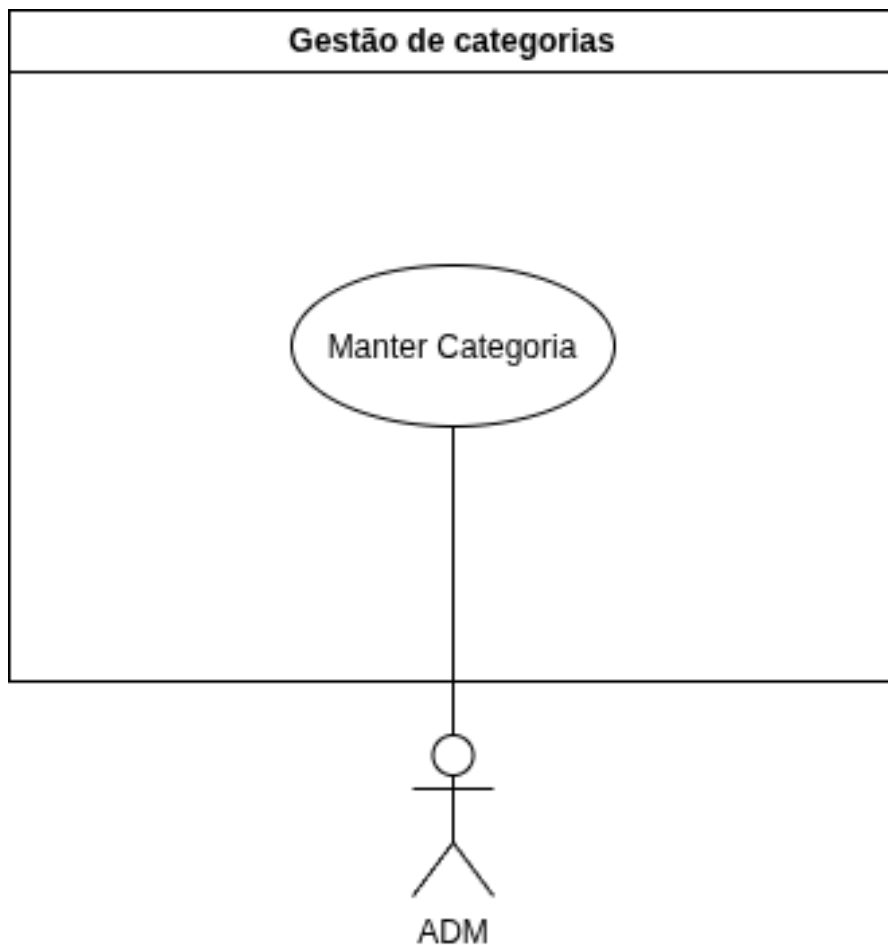
Figura 4 — Diagrama de casos de uso do módulo Gestão de Categorias
