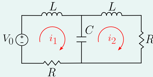
Figura 5.13: Circuito eléctrico.
