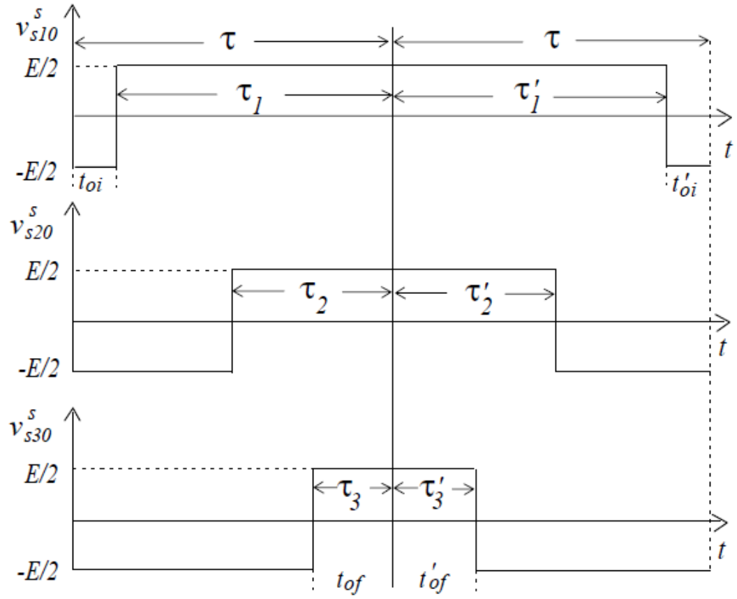
Figura 7.4: Tensões trifásicas para a modulação escalar.
