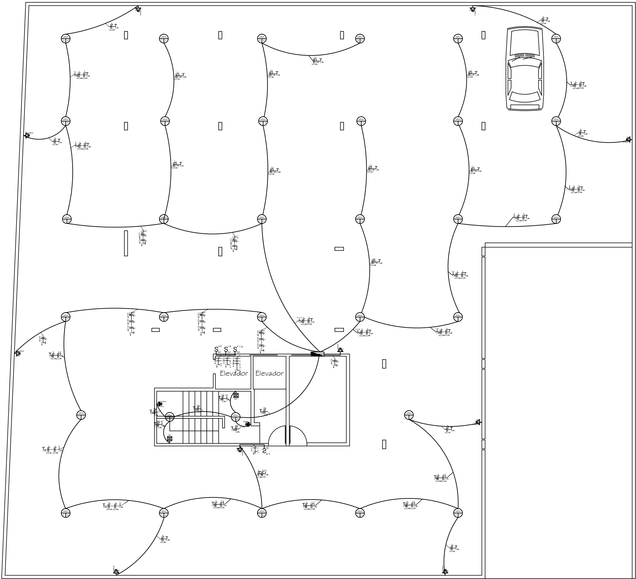
PLANTA DE SUBSOLO Escala _____ 1/50
