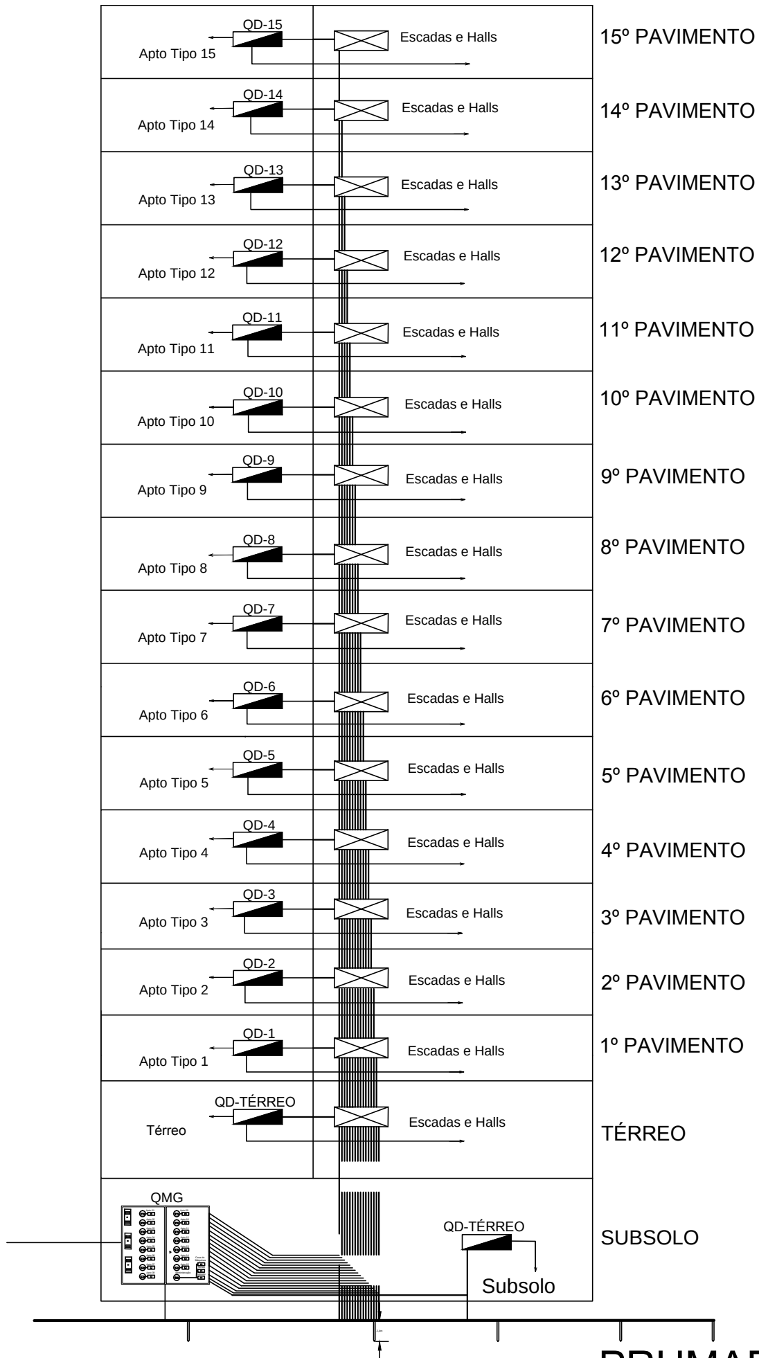
PRUMADA ELÉTRICA 1/50
