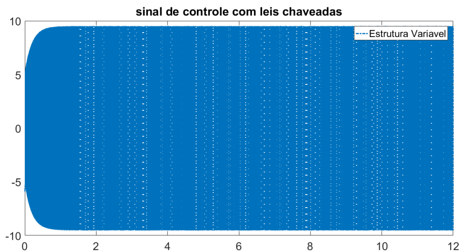
Figura 3.6: Sinal de controle para o controle adaptativo por modelo de referência e estrutura variável da planta de ordem 1, 12 segundos de simulação
