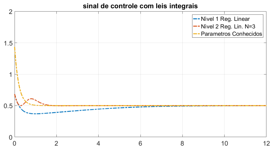
Figura 3.5: Sinal de controle para controle adaptativo indireto baseado no modelo de identificação por regressão linear, controle adaptativo indireto baseado em adaptação de segundo nível com N=3 e controle com parâmetros conhecidos da planta de ordem 1, 12 segundos de simulação
