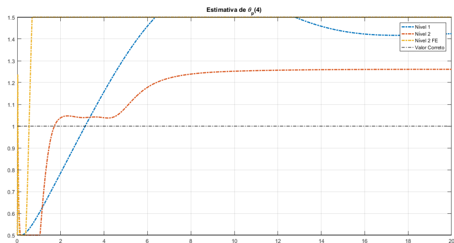
Figura 5.12: Comportamento das estimativas do coeficiente b_2 do polinômio N_p(s) para o modelo de primeiro nível, adaptação de segundo nível sem fator de esquecimento e adaptação de segundo nível com fator de esquecimento com referência degrau.
