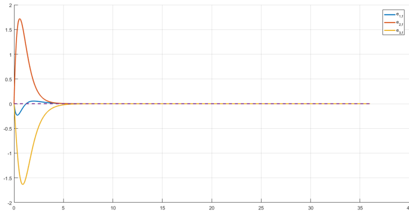
Figura 2.4: Erros de identificação usando 3 modelos por regressão linear para a planta \Sigma_p
