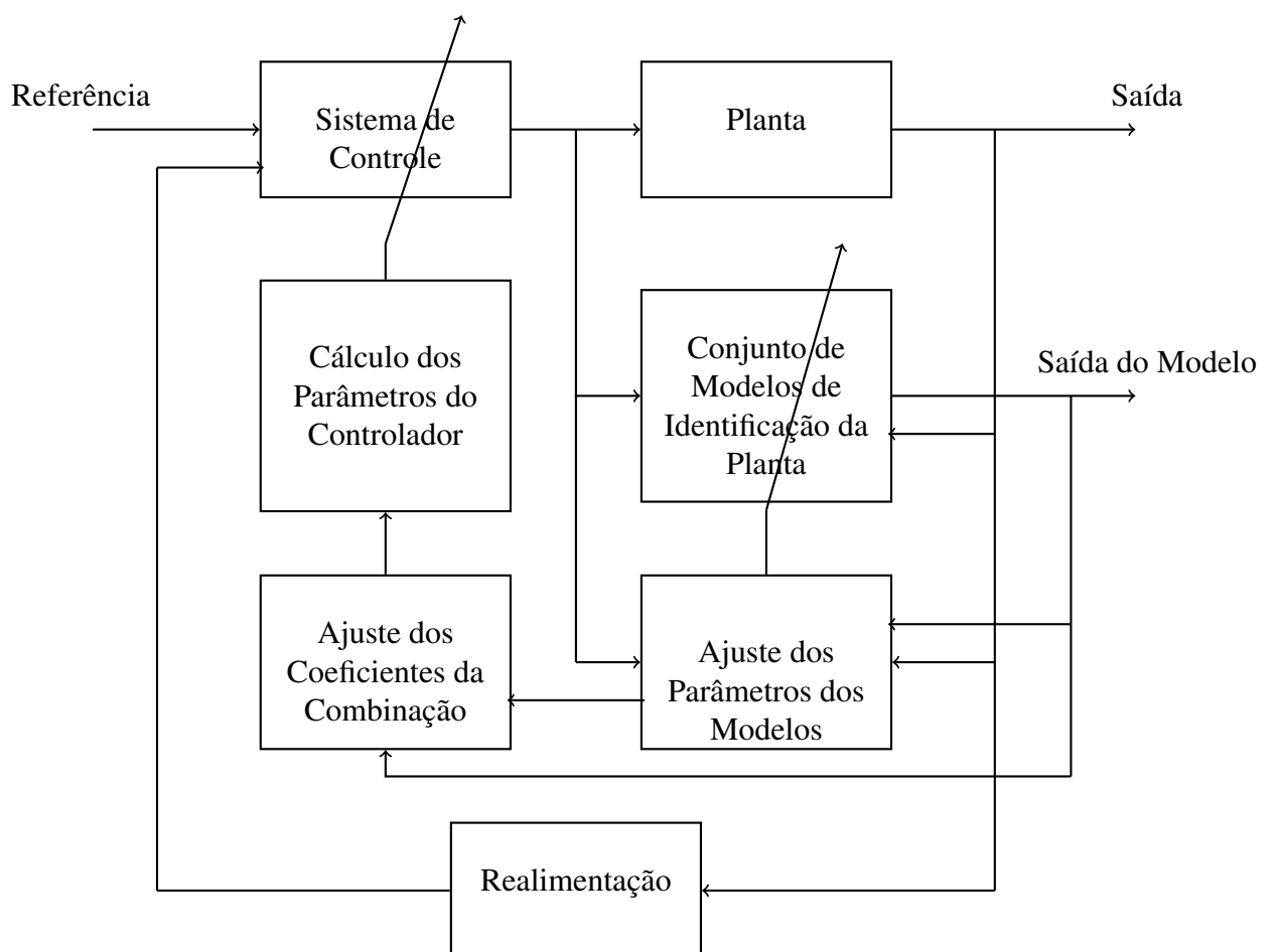
Figura 1.6: Controlador adaptativo indireto de segundo nível
