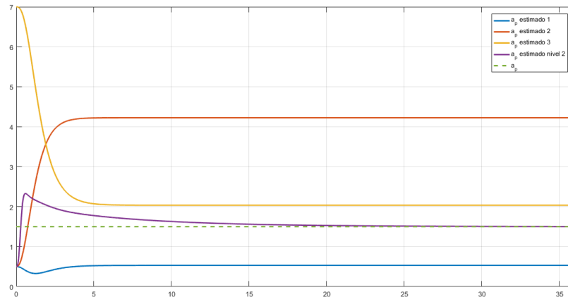
Figura 2.5: Estimativas do parâmetro a_p = 1.5 para a planta \Sigma_p para 3 modelos por regressão linear e a estimativa de segundo nível modificada, 36 segundos de simulação
