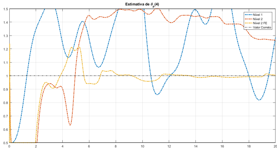
Figura 5.4: Comportamento das estimativas do coeficiente b_2 do polinômio N_p(s) para o modelo de primeiro nível, adaptação de segundo nível sem fator de esquecimento e adaptação de segundo nível com fator de esquecimento.
