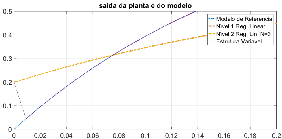
Figura 3.4: Detalhe da Figura 3.3, entre 0 e 0.2 segundos de simulação
