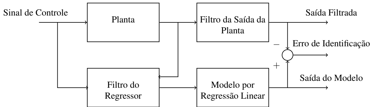
Figura 1.5: Modelo de identificação por regressão linear
