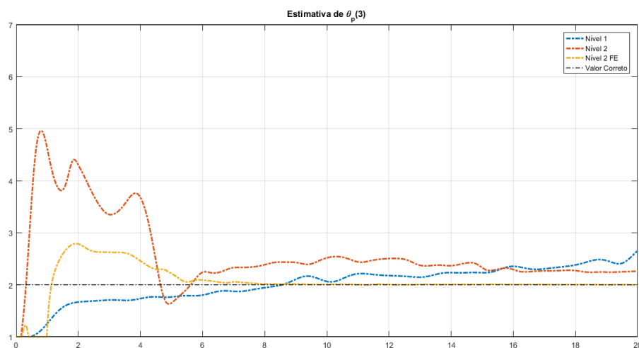
Figura 5.3: Comportamento das estimativas do coeficiente b_1 do polinômio N_p(s) para o modelo de primeiro nível, adaptação de segundo nível sem fator de esquecimento e adaptação de segundo nível com fator de esquecimento.
