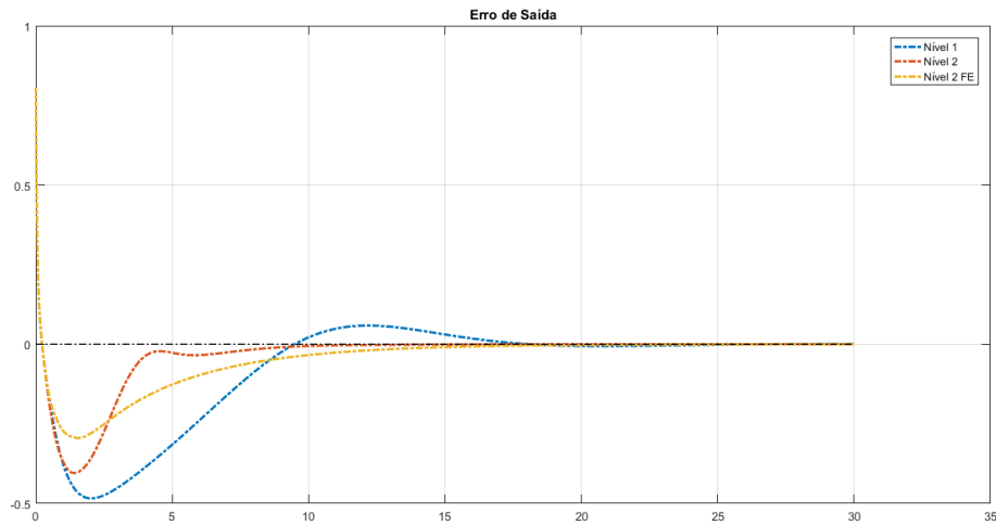
Figura 5.13: Erro de saída da planta para o modelo de primeiro nível, adaptação de segundo nível sem fator de esquecimento e adaptação de segundo nível com fator de esquecimento com referência degrau.
