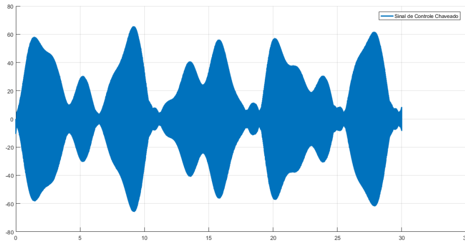
Figura 5.8: Sinal de controle gerado pelo controlador por modelo de referência e estrutura variável.
