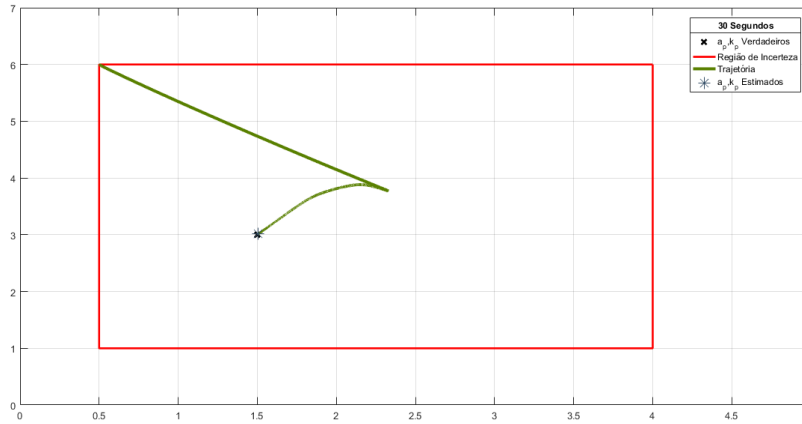
Figura 2.7: Trajetória dos parâmetros \hat{a}_{n2,f} e \hat{k}_{n2,f} da adaptação de segundo nível modificada no espaço de parâmetros usando 3 modelos por regressão linear para a planta \Sigma_p , aos 30 segundos de simulação
