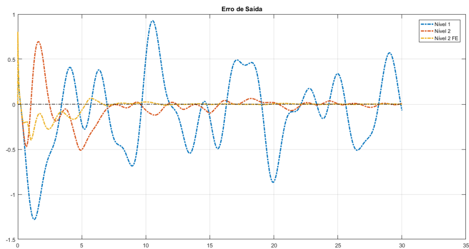
Figura 5.5: Erro de saída da planta para o modelo de primeiro nível, adaptação de segundo nível sem fator de esquecimento e adaptação de segundo nível com fator de esquecimento.
