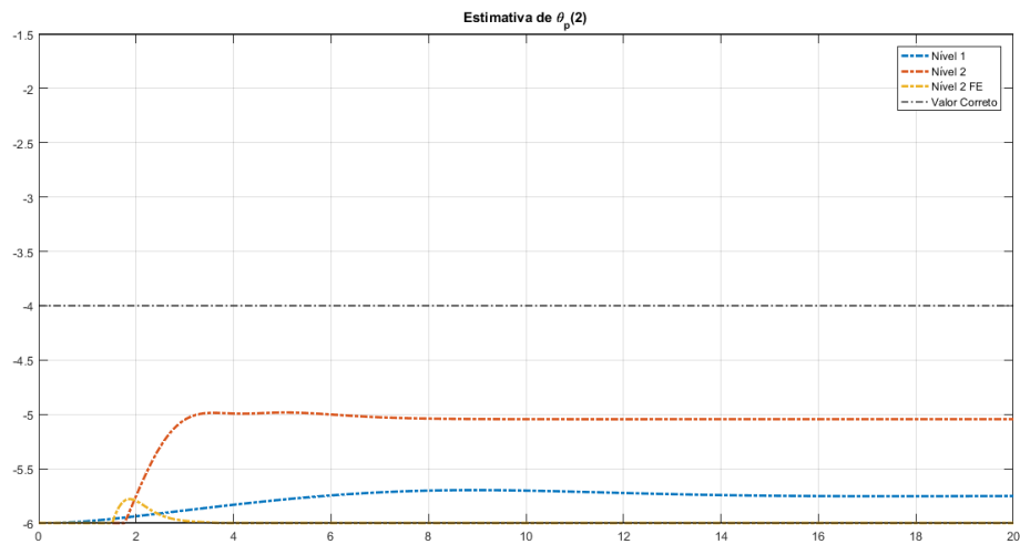
Figura 5.10: Comportamento das estimativas do coeficiente a_2 do polinômio D_p(s) para o modelo de primeiro nível, adaptação de segundo nível sem fator de esquecimento e adaptação de segundo nível com fator de esquecimento com referência degrau.
