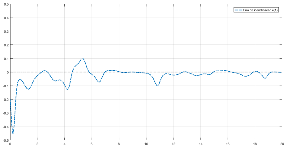
Figura 4.5: Erro de identificação não normalizado do modelo de primeiro nível com estimativa inicial \hat{\theta}_{1,f}(0) .
