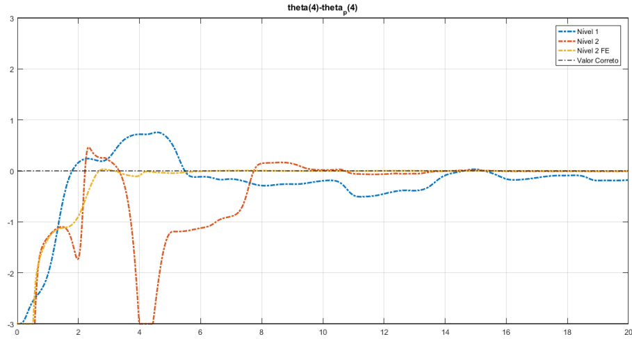
Figura 4.4: Comportamento das estimativas do coeficiente b_2 do polinômio N_p(s) para o modelo de primeiro nível, adaptação de segundo nível sem fator de esquecimento e adaptação de segundo nível com fator de esquecimento.
