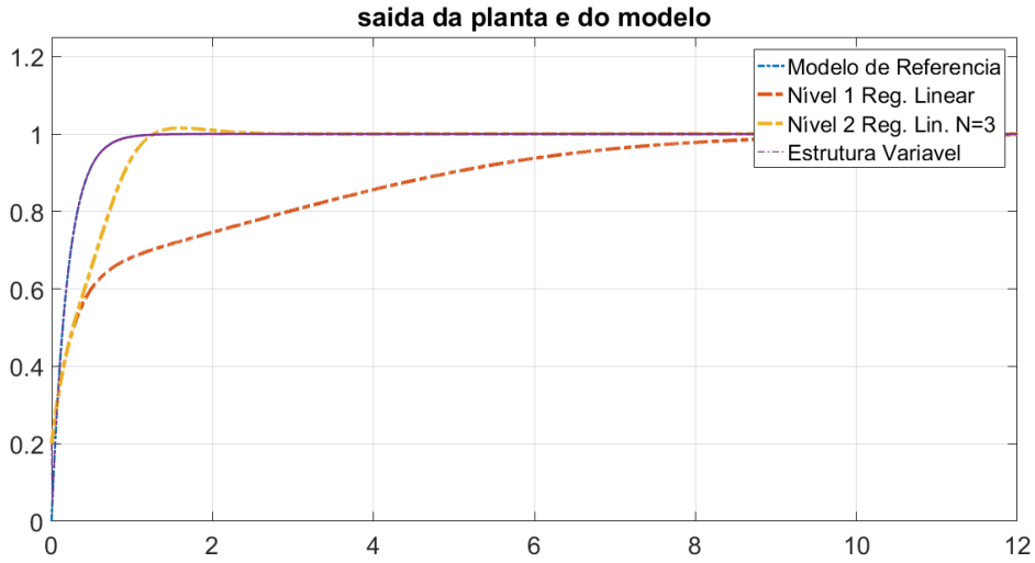
Figura 3.3: Saída da planta \Sigma_p de ordem 1 para o controle adaptativo indireto baseado no modelo de identificação por regressão linear, controle adaptativo indireto baseado em adaptação de segundo nível com N=3 , controle com estrutura variável e controle com parâmetros conhecidos, 12 segundos de simulação
