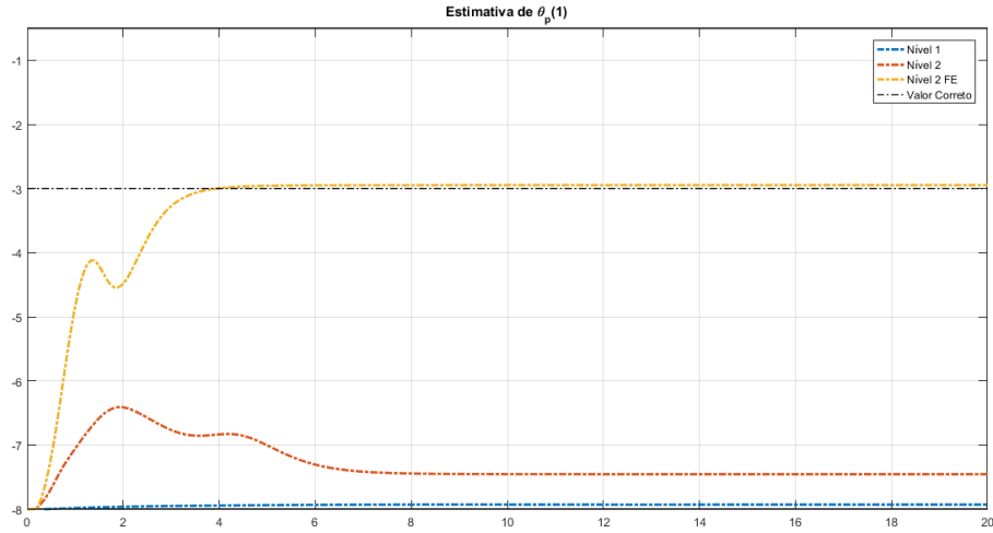
Figura 5.9: Comportamento das estimativas do coeficiente a_1 do polinômio D_p(s) para o modelo de primeiro nível, adaptação de segundo nível sem fator de esquecimento e adaptação de segundo nível com fator de esquecimento com referência degrau.
