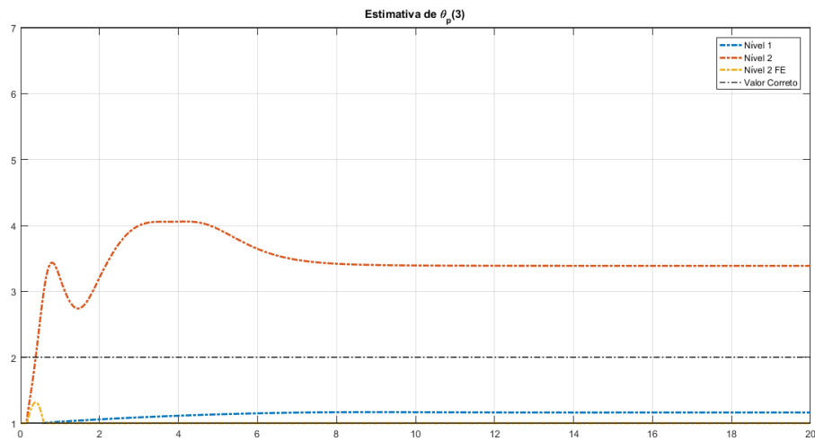
Figura 5.11: Comportamento das estimativas do coeficiente b_1 do polinômio N_p(s) para o modelo de primeiro nível, adaptação de segundo nível sem fator de esquecimento e adaptação de segundo nível com fator de esquecimento com referência degrau.
