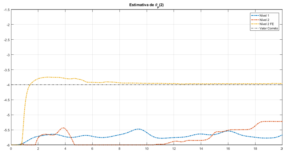
Figura 5.2: Comportamento das estimativas do coeficiente a_2 do polinômio D_p(s) para o modelo de primeiro nível, adaptação de segundo nível sem fator de esquecimento e adaptação de segundo nível com fator de esquecimento.
