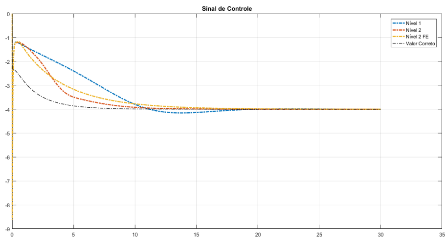
Figura 5.14: Sinal de controle gerado pelo controlador com base nas estimativas do modelo de primeiro nível, adaptação de segundo nível sem fator de esquecimento e adaptação de segundo nível com fator de esquecimento com referência degrau.
