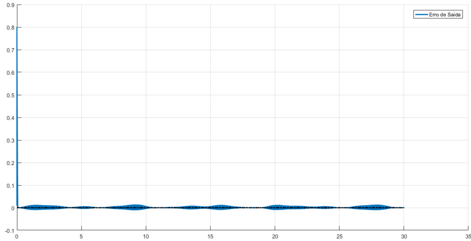
Figura 5.7: Erro de saída da planta para o controle por modelo de referência e estrutura variável.
