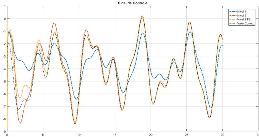
Figura 5.6: Sinal de controle gerado pelo controlador com base nas estimativas do modelo de primeiro nível, adaptação de segundo nível sem fator de esquecimento e adaptação de segundo nível com fator de esquecimento.
