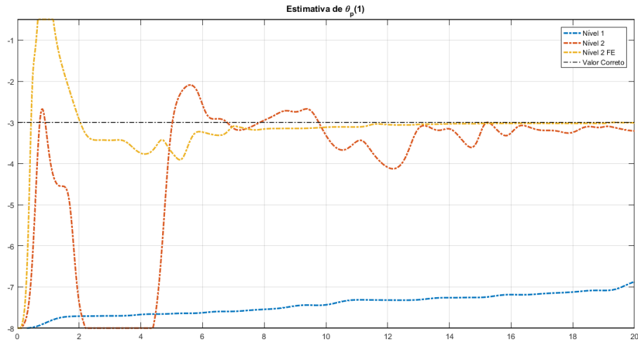
Figura 5.1: Comportamento das estimativas do coeficiente a_1 do polinômio D_p(s) para o modelo de primeiro nível, adaptação de segundo nível sem fator de esquecimento e adaptação de segundo nível com fator de esquecimento.
