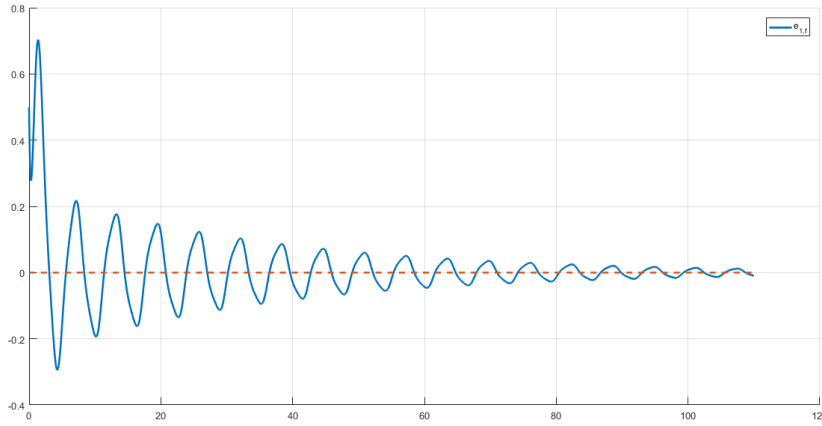
Figura 2.1: Erro de identificação usando o modelo por regressão linear para a planta \Sigma_p , 110 segundos de simulação
