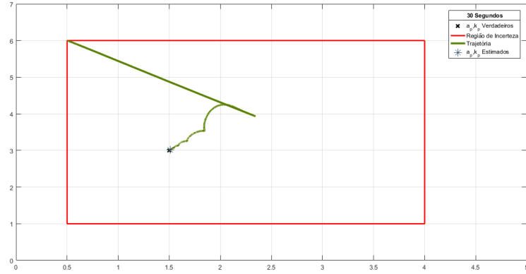
Figura 1.20: Trajetória dos parâmetros \hat{a}_{n2,sp} e \hat{k}_{n2,sp} da Adaptação de Segundo Nível no espaço de parâmetros usando 3 Modelos Série-Paralelo para a planta \Sigma_p , com função de transferência G(s) = \frac{3}{s+1.5} , com parâmetros iniciais dos Modelos \hat{a}_{1,sp}(0) = 0.5 e \hat{k}_{1,sp}(0) = 1 , \hat{a}_{2,sp}(0) = 0.5 e \hat{k}_{2,sp}(0) = 11 , \hat{a}_{3,sp}(0) = 7 e \hat{k}_{3,sp}(0) = 1 , e valores iniciais dos coeficientes \alpha_{1,sp}(0) = 0.5 , \alpha_{2,sp}(0) = 0.5 e \alpha_{3,sp}(0) = 0 , com a_m = 4 , para um passo de integração fixo de 10^{-3} segundos e 36 segundos de simulação
