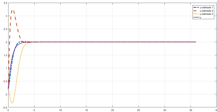
Figura 1.37: Saída da Planta e Estimativas da Saída da Planta usando Modelos Série-Paralelo para a planta \Sigma_p , com função de transferência G(s) = \frac{3}{s+1.5} , com parâmetros iniciais do Modelos \hat{a}_{1,sp}(0) = 0.5 e \hat{k}_{1,sp}(0) = 1 , \hat{a}_{2,sp}(0) = 0.5 e \hat{k}_{2,sp}(0) = 11 , \hat{a}_{3,sp}(0) = 7 e \hat{k}_{3,sp}(0) = 1 , com a_m = 4 , para um passo de integração fixo de 10^{-3} segundos e 36 segundos de simulação
