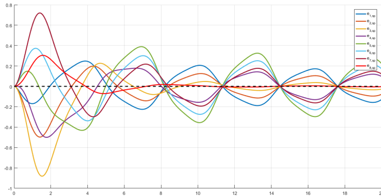
Figura 1.31: Erros de Identificação usando Modelos por Filtragem para a planta \Sigma_p , com função de transferência G(s) = \frac{3}{s+1.5} , com parâmetros iniciais dos Modelos \hat{a}_{1,f}(0) = 0.5 e \hat{k}_{1,f}(0) = 1 , \hat{a}_{2,f}(0) = 2.25 e \hat{k}_{2,f}(0) = 1 , \hat{a}_{3,f}(0) = 4 e \hat{k}_{3,f}(0) = 1 , \hat{a}_{4,f}(0) = 4 e \hat{k}_{4,f}(0) = 3.5 , \hat{a}_{5,f}(0) = 4 e \hat{k}_{5,f}(0) = 6 , \hat{a}_{6,f}(0) = 2.25 e \hat{k}_{6,f}(0) = 6 , \hat{a}_{7,f}(0) = 0.5 e \hat{k}_{7,f}(0) = 6 , \hat{a}_{8,f}(0) = 0.5 e \hat{k}_{8,f}(0) = 3.5 , com \lambda = 4 , para um passo de integração fixo de 10^{-3} segundos e 20 segundos de simulação
