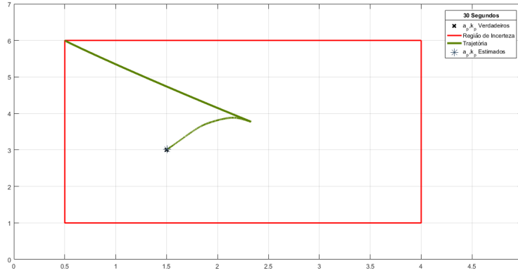
Figura 1.45: Trajetória dos parâmetros \hat{a}_{n2,f} e \hat{k}_{n2,f} da Adaptação de Segundo Nível Modificada no espaço de parâmetros usando 3 Modelos Série-Paralelo para a planta \Sigma_p , com função de transferência G(s) = \frac{3}{s+1.5} , com parâmetros iniciais dos Modelos \hat{a}_{1,f}(0) = 0.5 e \hat{k}_{1,f}(0) = 1 , \hat{a}_{2,f}(0) = 0.5 e \hat{k}_{2,f}(0) = 11 , \hat{a}_{3,f}(0) = 7 e \hat{k}_{3,f}(0) = 1 , e valores iniciais dos coeficientes \alpha_{1,f}(0) = 0.5 , \alpha_{2,f}(0) = 0.5 e \alpha_{3,f}(0) = 0 , com \lambda = 4 e u(t) = 1 , para um passo de integração fixo de 10^{-3} segundos e 36 segundos de simulação
