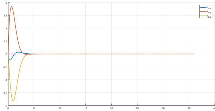
Figura 1.36: Erros de Identificação usando Modelos Série-Paralelo para a planta \Sigma_p , com função de transferência G(s) = \frac{3}{s+1.5} , com parâmetros iniciais dos Modelos \hat{a}_{1,sp}(0) = 0.5 e \hat{k}_{1,sp}(0) = 1 , \hat{a}_{2,sp}(0) = 0.5 e \hat{k}_{2,sp}(0) = 11 , \hat{a}_{3,sp}(0) = 7 e \hat{k}_{3,sp}(0) = 1 , com a_m = 4 , para um passo de integração fixo de 10^{-3} segundos e 36 segundos de simulação
