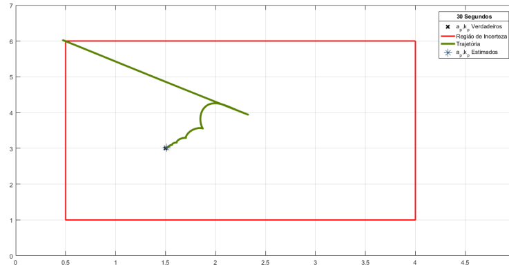
Figura 1.25: Trajetória dos parâmetros \hat{a}_{n2,f} e \hat{k}_{n2,f} da Adaptação de Segundo Nível no espaço de parâmetros usando 3 Modelos Série-Paralelo para a planta \Sigma_p , com função de transferência G(s) = \frac{3}{s+1.5} , com parâmetros iniciais dos Modelos \hat{a}_{1,f}(0) = 0.5 e \hat{k}_{1,f}(0) = 1, \hat{a}_{2,f}(0) = 0.5 e \hat{k}_{2,f}(0) = 11, \hat{a}_{3,f}(0) = 7 e \hat{k}_{3,f}(0) = 1 , e valores iniciais dos coeficientes \alpha_{1,sp}(0) = 0.5, \alpha_{2,sp}(0) = 0.5 e \alpha_{3,sp}(0) = 0 , com \lambda = 4 , para um passo de integração fixo de 10^{-3} segundos e 36 segundos de simulação
