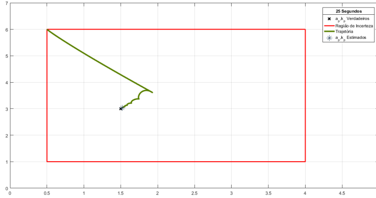
Figura 1.30: Trajetória dos parâmetros \hat{a}_{n2,f} e \hat{k}_{n2,f} da Adaptação de Segundo Nível no espaço de parâmetros usando 3 Modelos Série-Paralelo para a planta \Sigma_p , com função de transferência G(s) = \frac{3}{s+1.5} , com parâmetros iniciais dos Modelos \hat{a}_{1,f}(0) = 0.5 e \hat{k}_{1,f}(0) = 1 , \hat{a}_{2,f}(0) = 0.5 e \hat{k}_{2,f}(0) = 11 , \hat{a}_{3,f}(0) = 7 e \hat{k}_{3,f}(0) = 1 , e valores iniciais dos coeficientes \alpha_{1,sp}(0) = 0.5 , \alpha_{2,sp}(0) = 0.5 e \alpha_{3,sp}(0) = 0 , com \lambda = 4 , para um passo de integração fixo de 10^{-3} segundos e 25 segundos de simulação
