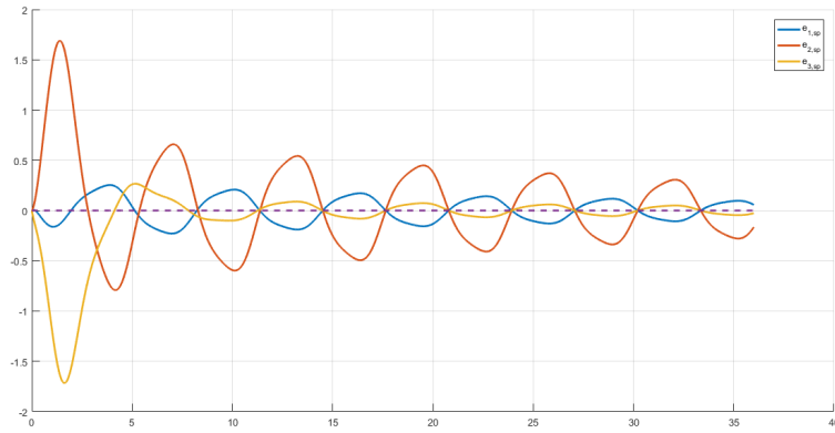
Figura 1.16: Erros de Identificação usando Modelos Série-Paralelo para a planta \Sigma_p , com função de transferência G(s) = \frac{3}{s+1.5} , com parâmetros iniciais dos Modelos \hat{a}_{1,sp}(0) = 0.5 e \hat{k}_{1,sp}(0) = 1 , \hat{a}_{2,sp}(0) = 0.5 e \hat{k}_{2,sp}(0) = 11 , \hat{a}_{3,sp}(0) = 7 e \hat{k}_{3,sp}(0) = 1 , com a_m = 4 , para um passo de integração fixo de 10^{-3} segundos e 36 segundos de simulação
