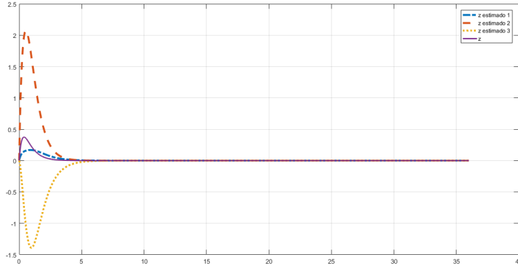
Figura 1.42: Saída da Planta e Estimativas da Saída da Planta usando Modelos por Filtragem para a planta \Sigma_p , com função de transferência G(s) = \frac{3}{s+1.5} , com parâmetros iniciais dos Modelos \hat{a}_{1,f}(0) = 0.5 e \hat{k}_{1,f}(0) = 1 , \hat{a}_{2,f}(0) = 0.5 e \hat{k}_{2,f}(0) = 11 , \hat{a}_{3,f}(0) = 7 e \hat{k}_{3,f}(0) = 1 , com \lambda = 4 e u(t) = 1 , para um passo de integração fixo de 10^{-3} segundos e 36 segundos de simulação
