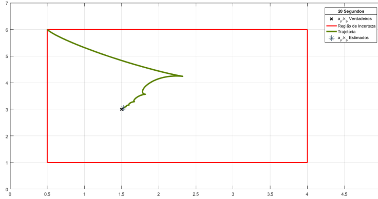
Figura 1.35: Trajetória dos parâmetros \hat{a}_{n2,f} e \hat{k}_{n2,f} da Adaptação de Segundo Nível no espaço de parâmetros usando 3 Modelos Série-Paralelo para a planta \Sigma_p , com função de transferência G(s) = \frac{3}{s+1.5} , com parâmetros iniciais dos Modelos \hat{a}_{1,f}(0) = 0.5 e \hat{a}_{1,f}(0) = 0.5 e \hat{k}_{1,f}(0) = 1 , \hat{a}_{2,f}(0) = 2.25 e \hat{k}_{2,f}(0) = 1 , \hat{a}_{3,f}(0) = 4 e \hat{k}_{3,f}(0) = 1 , \hat{a}_{3,f}(0) = 4 e \hat{k}_{3,f}(0) = 1 , \hat{a}_{4,f}(0) = 4 e \hat{k}_{4,f}(0) = 3.5 , \hat{a}_{5,f}(0) = 4 e \hat{k}_{5,f}(0) = 6 , \hat{a}_{6,f}(0) = 2.25 e \hat{k}_{6,f}(0) = 6 , \hat{a}_{7,f}(0) = 0.5 e \hat{k}_{7,f}(0) = 6 , \hat{a}_{8,f}(0) = 0.5 e \hat{k}_{8,f}(0) = 3.5 , e valor inicial dos coeficiente \alpha_{7,sp}(0) = 1 , com os demais coeficientes iguais a zero inicialmente, com \lambda = 4 , para um passo de integração fixo de 10^{-3} segundos e 20 segundos de simulação
