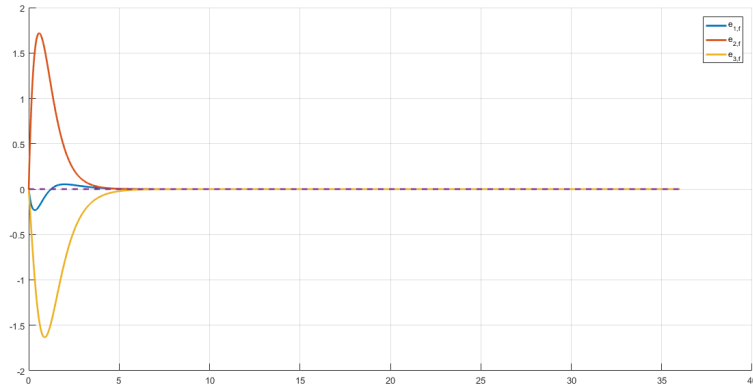
Figura 1.41: Erros de Identificação usando Modelos por Filtragem para a planta \Sigma_p , com função de transferência G(s) = \frac{3}{s+1.5} , com parâmetros iniciais dos Modelos \hat{a}_{1,f}(0) = 0.5 e \hat{k}_{1,f}(0) = 1 , \hat{a}_{2,f}(0) = 0.5 e \hat{k}_{2,f}(0) = 11 , \hat{a}_{3,f}(0) = 7 e \hat{k}_{3,f}(0) = 1 , com \lambda = 4 e u(t) = 1 , para um passo de integração fixo de 10^{-3} segundos e 36 segundos de simulação
