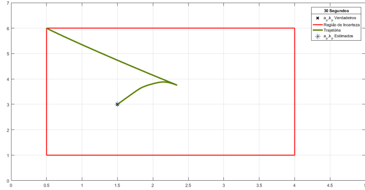
Figura 1.40: Trajetória dos parâmetros \hat{a}_{n2,sp} e \hat{k}_{n2,sp} da Adaptação de Segundo Nível no espaço de parâmetros usando 3 Modelos Série-Paralelo para a planta \Sigma_p , com função de transferência G(s) = \frac{3}{s+1.5} , com parâmetros iniciais dos Modelos \hat{a}_{1,sp}(0) = 0.5 e \hat{k}_{1,sp}(0) = 1 , \hat{a}_{2,sp}(0) = 0.5 e \hat{k}_{2,sp}(0) = 11 , \hat{a}_{3,sp}(0) = 7 e \hat{k}_{3,sp}(0) = 1 , e valores iniciais dos coeficientes \alpha_{1,sp}(0) = 0.5 , \alpha_{2,sp}(0) = 0.5 e \alpha_{3,sp}(0) = 0 , com a_m = 4 , para um passo de integração fixo de 10^{-3} segundos e 36 segundos de simulação
