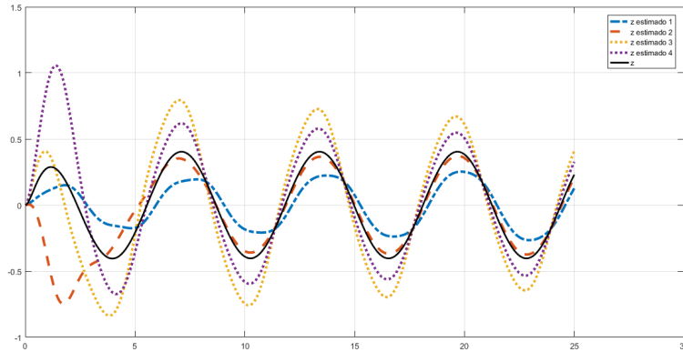
Figura 1.27: Saída da Planta e Estimativas da Saída da Planta usando Modelos por Filtragem para a planta \Sigma_p , com função de transferência G(s) = \frac{3}{s+1.5} , com parâmetros iniciais do Modelos \hat{a}_{1,f}(0) = 0.5 e \hat{k}_{1,f}(0) = 1 , \hat{a}_{2,f}(0) = 0.5 e \hat{k}_{2,f}(0) = 11 , \hat{a}_{3,f}(0) = 7 e \hat{k}_{3,f}(0) = 1 , com \lambda = 4 , para um passo de integração fixo de 10^{-3} segundos e 25 segundos de simulação
