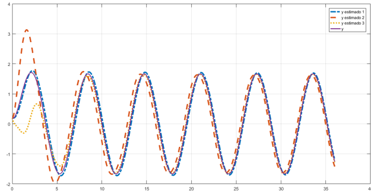
Figura 1.17: Saída da Planta e Estimativas da Saída da Planta usando Modelos Série-Paralelo para a planta \Sigma_p , com função de transferência G(s) = \frac{3}{s+1.5} , com parâmetros iniciais do Modelos \hat{a}_{1,sp}(0) = 0.5 e \hat{k}_{1,sp}(0) = 1 , \hat{a}_{2,sp}(0) = 0.5 e \hat{k}_{2,sp}(0) = 11 , \hat{a}_{3,sp}(0) = 7 e \hat{k}_{3,sp}(0) = 1 , com a_m = 4 , para um passo de integração fixo de 10^{-3} segundos e 36 segundos de simulação
