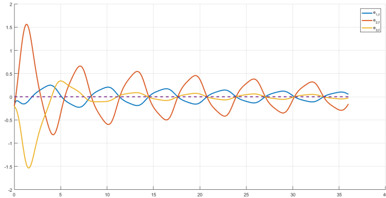
Figura 1.21: Erros de Identificação usando Modelos por Filtragem para a planta \Sigma_p , com função de transferência G(s) = \frac{3}{s+1.5} , com parâmetros iniciais dos Modelos \hat{a}_{1,f}(0) = 0.5 e \hat{k}_{1,f}(0) = 1 , \hat{a}_{2,f}(0) = 0.5 e \hat{k}_{2,f}(0) = 11 , \hat{a}_{3,f}(0) = 7 e \hat{k}_{3,f}(0) = 1 , com \lambda = 4 , para um passo de integração fixo de 10^{-3} segundos e 36 segundos de simulação
