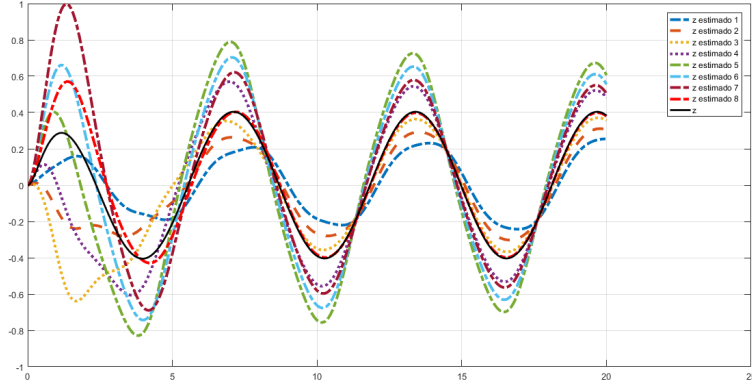
Figura 1.32: Saída da Planta e Estimativas da Saída da Planta usando Modelos por Filtragem para a planta \Sigma_p , com função de transferência G(s) = \frac{3}{s+1.5} , com parâmetros iniciais do Modelos \hat{a}_{1,f}(0) = 0.5 e \hat{k}_{1,f}(0) = 1 , \hat{a}_{2,f}(0) = 2.25 e \hat{k}_{2,f}(0) = 1 , \hat{a}_{3,f}(0) = 4 e \hat{k}_{3,f}(0) = 1 , \hat{a}_{3,f}(0) = 4 e \hat{k}_{3,f}(0) = 1 , \hat{a}_{4,f}(0) = 4 e \hat{k}_{4,f}(0) = 3.5 , \hat{a}_{5,f}(0) = 4 e \hat{k}_{5,f}(0) = 6 , \hat{a}_{6,f}(0) = 2.25 e \hat{k}_{6,f}(0) = 6 , \hat{a}_{7,f}(0) = 0.5 e \hat{k}_{7,f}(0) = 6 , \hat{a}_{8,f}(0) = 0.5 e \hat{k}_{8,f}(0) = 3.5 , com \lambda = 4 , para um passo de integração fixo de 10^{-3} segundos e 20 segundos de simulação
