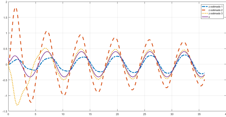
Figura 1.22: Saída da Planta e Estimativas da Saída da Planta usando Modelos por Filtragem para a planta \Sigma_p , com função de transferência G(s) = \frac{3}{s+1.5} , com parâmetros iniciais dos Modelos \hat{a}_{1,f}(0) = 0.5 e \hat{k}_{1,f}(0) = 1, \hat{a}_{2,f}(0) = 0.5 e \hat{k}_{2,f}(0) = 11, \hat{a}_{3,f}(0) = 7 e \hat{k}_{3,f}(0) = 1 , com \lambda = 4 , para um passo de integração fixo de 10^{-3} segundos e 36 segundos de simulação
