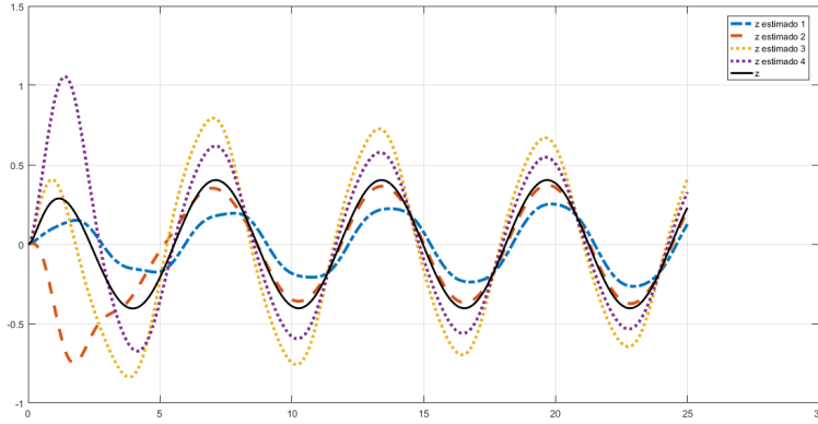
Figura 1.27: Saída da Planta e Estimativas da Saída da Planta usando Modelos por Filtragem para a planta \Sigma_p , com função de transferência G(s) = \frac{3}{s+1.5} , com parâmetros iniciais dos Modelos \hat{a}_{1,f}(0) = 0.5 e \hat{k}_{1,f}(0) = 1, \hat{a}_{2,f}(0) = 0.5 e \hat{k}_{2,f}(0) = 11, \hat{a}_{3,f}(0) = 7 e \hat{k}_{3,f}(0) = 1 , com \lambda = 4 , para um passo de integração fixo de 10^{-3} segundos e 25 segundos de simulação
