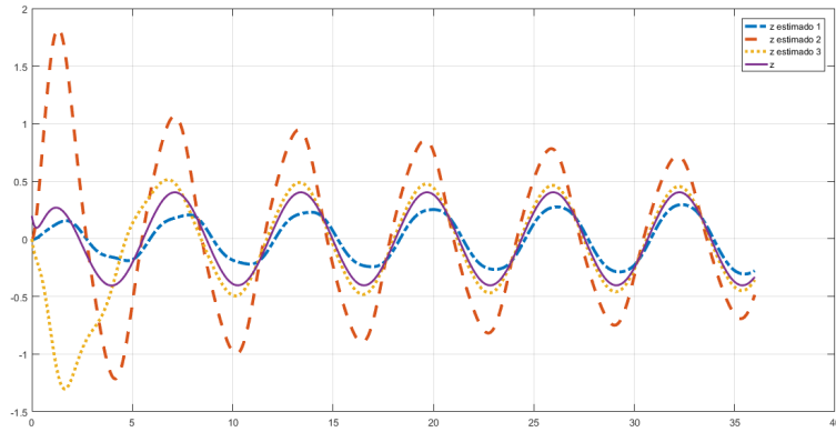
Figura 1.22: Saída da Planta e Estimativas da Saída da Planta usando Modelos por Filtragem para a planta \Sigma_p , com função de transferência G(s) = \frac{3}{s+1.5} , com parâmetros iniciais do Modelos \hat{a}_{1,f}(0) = 0.5 e \hat{k}_{1,f}(0) = 1, \hat{a}_{2,f}(0) = 0.5 e \hat{k}_{2,f}(0) = 11, \hat{a}_{3,f}(0) = 7 e \hat{k}_{3,f}(0) = 1 , com \lambda = 4 , para um passo de integração fixo de 10^{-3} segundos e 36 segundos de simulação
