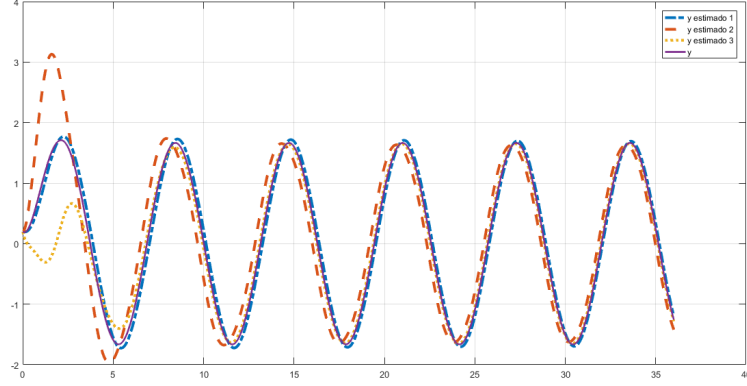
Figura 1.17: Saída da Planta e Estimativas da Saída da Planta usando Modelos Série-Paralelo para a planta \Sigma_p , com função de transferência G(s) = \frac{3}{s+1.5} , com parâmetros iniciais dos Modelos \hat{a}_{1,sp}(0) = 0.5 e \hat{k}_{1,sp}(0) = 1 , \hat{a}_{2,sp}(0) = 0.5 e \hat{k}_{2,sp}(0) = 11 , \hat{a}_{3,sp}(0) = 7 e \hat{k}_{3,sp}(0) = 1 , com a_m = 4 , para um passo de integração fixo de 10^{-3} segundos e 36 segundos de simulação
