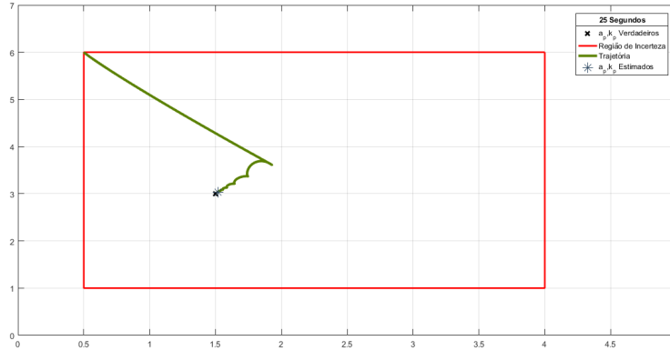
Figura 1.30: Trajetória dos parâmetros \hat{a}_{n2,f} e \hat{k}_{n2,f} da Adaptação de Segundo Nível no espaço de parâmetros usando 4 Modelos por Regressão Linear para a planta \Sigma_p , com função de transferência G(s) = \frac{3}{s+1.5} , com parâmetros iniciais dos Modelos \hat{a}_{1,f}(0) = 0.5 e \hat{k}_{1,f}(0) = 1 , \hat{a}_{2,f}(0) = 4 e \hat{k}_{2,f}(0) = 1 , \hat{a}_{3,f}(0) = 4 e \hat{k}_{3,f}(0) = 6 e \hat{a}_{4,f}(0) = 0.5 e \hat{k}_{4,f}(0) = 6 , e valores iniciais dos coeficientes \alpha_{1,f}(0) = 0 , \alpha_{2,f}(0) = 0 e \alpha_{3,f}(0) = 0 e \alpha_{4,f}(0) = 1 , com \lambda = 4 , para um passo de integração fixo de 10^{-3} segundos e 25 segundos de simulação
