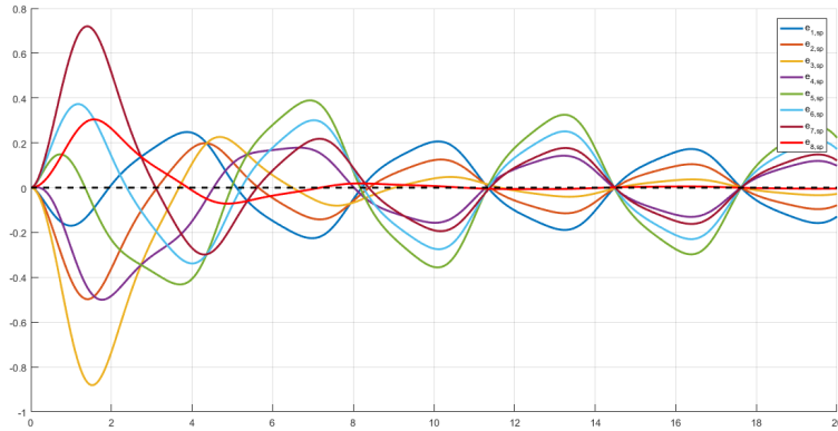
Figura 1.31: Erros de Identificação usando 8 Modelos por Regressão Linear para a planta \Sigma_p , com função de transferência G(s) = \frac{3}{s+1.5} , com parâmetros iniciais dos Modelos \hat{a}_{1,f}(0) = 0.5 e \hat{k}_{1,f}(0) = 1 , \hat{a}_{2,f}(0) = 2.25 e \hat{k}_{2,f}(0) = 1 , \hat{a}_{3,f}(0) = 4 e \hat{k}_{3,f}(0) = 1 , \hat{a}_{4,f}(0) = 4 e \hat{k}_{4,f}(0) = 3.5 , \hat{a}_{5,f}(0) = 4 e \hat{k}_{5,f}(0) = 6 , \hat{a}_{6,f}(0) = 2.25 e \hat{k}_{6,f}(0) = 6 , \hat{a}_{7,f}(0) = 0.5 e \hat{k}_{7,f}(0) = 6 , \hat{a}_{8,f}(0) = 0.5 e \hat{k}_{8,f}(0) = 3.5 , com \lambda = 4 , para um passo de integração fixo de 10^{-3} segundos e 20 segundos de simulação
