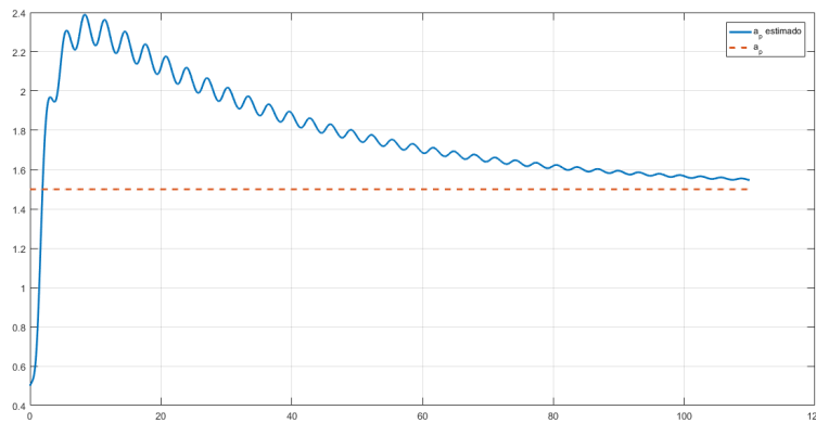
Figura 1.13: Estimativa do parâmetro a_p = 1.5 usando o Modelo por Regressão Linear para a planta \Sigma_p , com função de transferência G(s) = \frac{3}{s+1.5} , com parâmetros iniciais do Modelo \hat{a}_{1,f}(0) = 0.5 e \hat{k}_{1,f}(0) = 6 , com \lambda = 4 , para um passo de integração fixo de 10^{-3} segundos e 110 segundos de simulação
