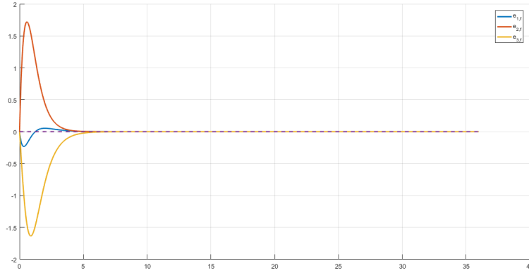
Figura 1.41: Erros de Identificação usando 3 Modelos por Regressão Linear para a planta \Sigma_p , com função de transferência G(s) = \frac{3}{s+1.5} , com parâmetros iniciais dos Modelos \hat{a}_{1,f}(0) = 0.5 e \hat{k}_{1,f}(0) = 1 , \hat{a}_{2,f}(0) = 0.5 e \hat{k}_{2,f}(0) = 11 , \hat{a}_{3,f}(0) = 7 e \hat{k}_{3,f}(0) = 1 , com \lambda = 4 e u(t) = 1 , para um passo de integração fixo de 10^{-3} segundos e 36 segundos de simulação
