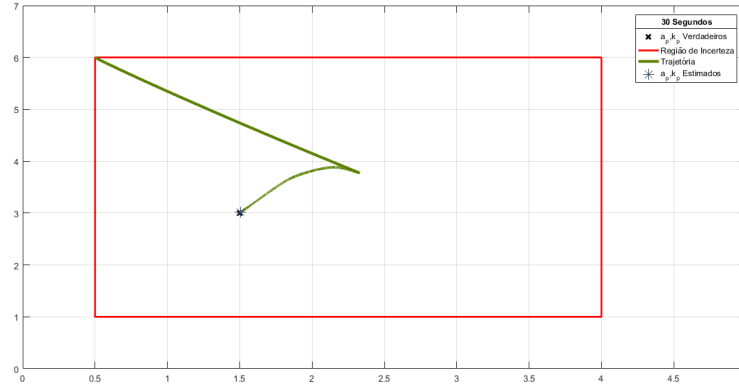
Figura 1.45: Trajetória dos parâmetros \hat{a}_{n2,f} e \hat{k}_{n2,f} da Adaptação de Segundo Nível Modificada no espaço de parâmetros usando 3 Modelos por Regressão Linear para a planta \Sigma_p , com função de transferência G(s) = \frac{3}{s+1.5} , com parâmetros iniciais dos Modelos \hat{a}_{1,f}(0) = 0.5 e \hat{k}_{1,f}(0) = 1 , \hat{a}_{2,f}(0) = 0.5 e \hat{k}_{2,f}(0) = 11 , \hat{a}_{3,f}(0) = 7 e \hat{k}_{3,f}(0) = 1 , e valores iniciais dos coeficientes \alpha_{1,f}(0) = 0.5 , \alpha_{2,f}(0) = 0.5 e \alpha_{3,f}(0) = 0 , com \lambda = 4 e u(t) = 1 , para um passo de integração fixo de 10^{-3} segundos e 36 segundos de simulação
