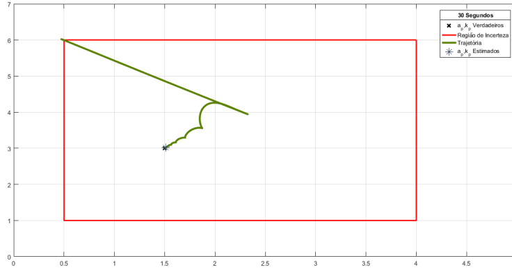
Figura 1.25: Trajetória dos parâmetros \hat{a}_{n2,f} e \hat{k}_{n2,f} da Adaptação de Segundo Nível no espaço de parâmetros usando 3 Modelos por Regressão Linear para a planta \Sigma_p , com função de transferência G(s) = \frac{3}{s+1.5} , com parâmetros iniciais dos Modelos \hat{a}_{1,f}(0) = 0.5 e \hat{k}_{1,f}(0) = 1 , \hat{a}_{2,f}(0) = 0.5 e \hat{k}_{2,f}(0) = 11 , \hat{a}_{3,f}(0) = 7 e \hat{k}_{3,f}(0) = 1 , e valores iniciais dos coeficientes \alpha_{1,sp}(0) = 0.5 , \alpha_{2,sp}(0) = 0.5 e \alpha_{3,sp}(0) = 0 , com \lambda = 4 , para um passo de integração fixo de 10^{-3} segundos e 36 segundos de simulação
