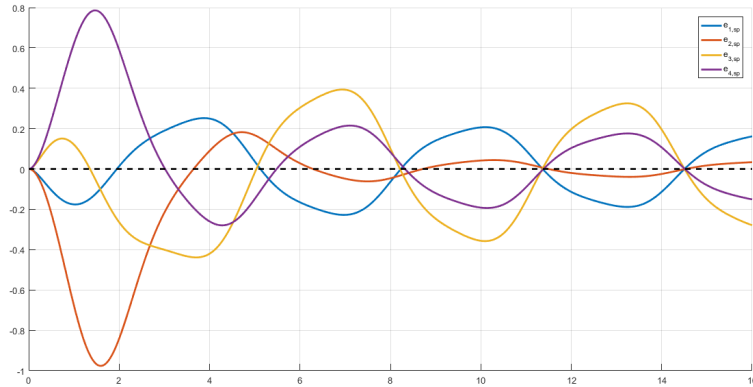
Figura 1.26: Erros de Identificação usando 4 Modelos por Regressão Linear para a planta \Sigma_p , com função de transferência G(s) = \frac{3}{s+1.5} , com parâmetros iniciais dos Modelos \hat{a}_{1,f}(0) = 0.5 e \hat{k}_{1,f}(0) = 1, \hat{a}_{2,f}(0) = 4 e \hat{k}_{2,f}(0) = 1, \hat{a}_{3,f}(0) = 4 e \hat{k}_{3,f}(0) = 6 e \hat{a}_{4,f}(0) = 0.5 e \hat{k}_{4,f}(0) = 6 , com \lambda = 4 , para um passo de integração fixo de 10^{-3} segundos e detalhe dos primeiros 16 segundos de simulação
