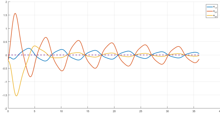
Figura 1.21: Erros de Identificação usando 3 Modelos por Regressão Linear para a planta \Sigma_p , com função de transferência G(s) = \frac{3}{s+1.5} , com parâmetros iniciais dos Modelos \hat{a}_{1,f}(0) = 0.5 e \hat{k}_{1,f}(0) = 1 , \hat{a}_{2,f}(0) = 0.5 e \hat{k}_{2,f}(0) = 11 , \hat{a}_{3,f}(0) = 7 e \hat{k}_{3,f}(0) = 1 , com \lambda = 4 , para um passo de integração fixo de 10^{-3} segundos e 36 segundos de simulação
