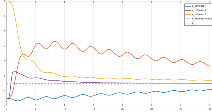
Figura 1.23: Estimativas do parâmetro a_p = 1.5 para a planta \Sigma_p para 3 Modelos por Regressão Linear e a estimativa de Segundo Nível entregue pela combinação convexa de coeficientes \alpha_{1,f}, \alpha_{2,f} e \alpha_{3,f} destas estimativas, com função de transferência G(s) = \frac{3}{s+1.5} , com parâmetros iniciais dos Modelos \hat{a}_{1,f}(0) = 0.5 e \hat{k}_{1,f}(0) = 1, \hat{a}_{2,f}(0) = 0.5 e \hat{k}_{2,f}(0) = 11, \hat{a}_{3,f}(0) = 7 e \hat{k}_{3,f}(0) = 1 , e valores iniciais dos coeficientes \alpha_{1,f}(0) = 0.5, \alpha_{2,f}(0) = 0.5 e \alpha_{3,f}(0) = 0 , com \lambda = 4 , para um passo de integração fixo de 10^{-3} segundos e 36 segundos de simulação
