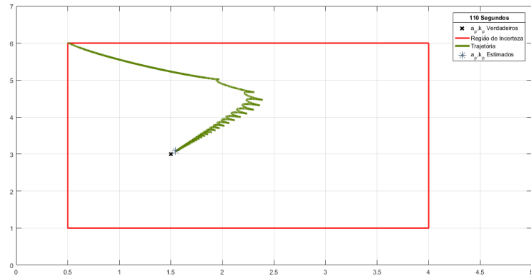
Figura 1.15: Trajetória dos parâmetros \hat{a}_{1,f} e \hat{k}_{1,f} no espaço de parâmetros usando o Modelo por Regressão Linear para a planta \Sigma_p , com função de transferência G(s) = \frac{3}{s+1.5} , com parâmetros iniciais do Modelo \hat{a}_{1,f}(0) = 0.5 e \hat{k}_{1,f}(0) = 6 , com \lambda = 4 , para um passo de integração fixo de 10^{-3} segundos e 110 segundos de simulação
