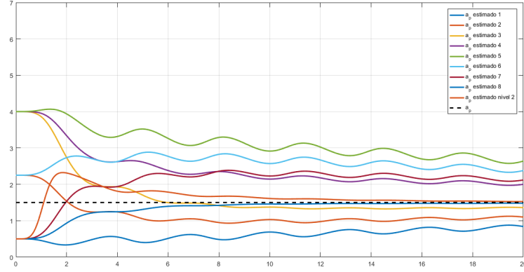
Figura 1.33: Estimativas do parâmetro a_p = 1.5 para a planta \Sigma_p para 8 Modelos por Regressão Linear e a estimativa de Segundo Nível entregue pela combinação convexa de coeficientes \alpha_{1,f}, \alpha_{2,f}, \alpha_{3,f}, \alpha_{4,f}, \alpha_{5,f}, \alpha_{6,f}, \alpha_{7,f} e \alpha_{8,f} destas estimativas, com função de transferência G(s) = \frac{3}{s+1.5} , com parâmetros iniciais dos Modelos \hat{a}_{1,f}(0) = 0.5 e \hat{k}_{1,f}(0) = 1, \hat{a}_{2,f}(0) = 2.25 e \hat{k}_{2,f}(0) = 1, \hat{a}_{3,f}(0) = 4 e \hat{k}_{3,f}(0) = 1, \hat{a}_{4,f}(0) = 4 e \hat{k}_{4,f}(0) = 3.5, \hat{a}_{5,f}(0) = 4 e \hat{k}_{5,f}(0) = 6, \hat{a}_{6,f}(0) = 2.25 e \hat{k}_{6,f}(0) = 6, \hat{a}_{7,f}(0) = 0.5 e \hat{k}_{7,f}(0) = 6, \hat{a}_{8,f}(0) = 0.5 e \hat{k}_{8,f}(0) = 3.5 , e valor inicial de \alpha_{7,sp}(0) = 1 , com os demais coeficientes iguais a zero inicialmente, com \lambda = 4 , para um passo de integração fixo de 10^{-3} segundos e 20 segundos de simulação
