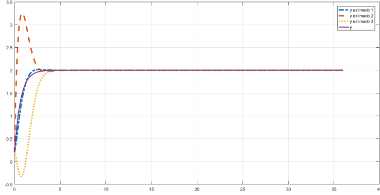
Figura 1.37: Saída da Planta e Estimativas da Saída da Planta usando 3 Modelos Série-Paralelos para a planta \Sigma_p , com função de transferência G(s) = \frac{3}{s+1.5} , com parâmetros iniciais dos Modelos \hat{a}_{1,sp}(0) = 0.5 e \hat{k}_{1,sp}(0) = 1 , \hat{a}_{2,sp}(0) = 0.5 e \hat{k}_{2,sp}(0) = 11 , \hat{a}_{3,sp}(0) = 7 e \hat{k}_{3,sp}(0) = 1 , com a_m = 4 , para um passo de integração fixo de 10^{-3} segundos e 36 segundos de simulação
