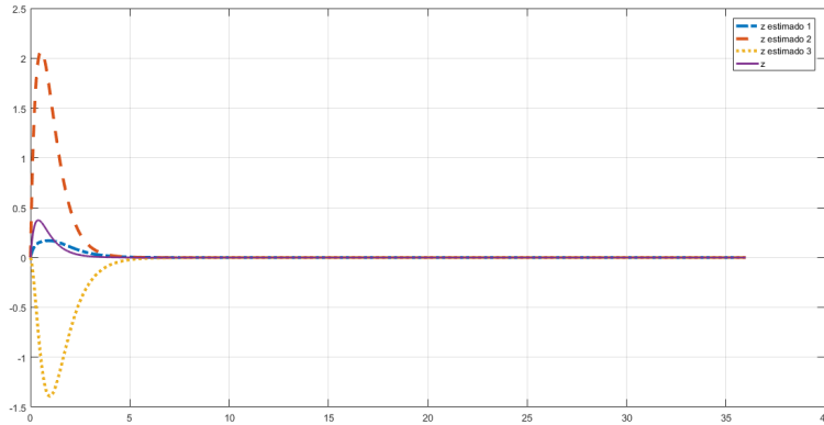
Figura 1.42: Saída da Planta e Estimativas da Saída da Planta usando 3 Modelos por Regressão Linear para a planta \Sigma_p , com função de transferência G(s) = \frac{3}{s+1.5} , com parâmetros iniciais do Modelos \hat{a}_{1,f}(0) = 0.5 e \hat{k}_{1,f}(0) = 1 , \hat{a}_{2,f}(0) = 0.5 e \hat{k}_{2,f}(0) = 11 , \hat{a}_{3,f}(0) = 7 e \hat{k}_{3,f}(0) = 1 , com \lambda = 4 e u(t) = 1 , para um passo de integração fixo de 10^{-3} segundos e 36 segundos de simulação
