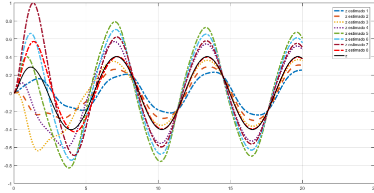
Figura 1.32: Saída da Planta e Estimativas da Saída da Planta usando 8 Modelos por Regressão Linear para a planta \Sigma_p , com função de transferência G(s) = \frac{3}{s+1.5} , com parâmetros iniciais dos Modelos \hat{a}_{1,f}(0) = 0.5 e \hat{k}_{1,f}(0) = 1 , \hat{a}_{2,f}(0) = 2.25 e \hat{k}_{2,f}(0) = 1 , \hat{a}_{3,f}(0) = 4 e \hat{k}_{3,f}(0) = 1 , \hat{a}_{3,f}(0) = 4 e \hat{k}_{3,f}(0) = 1 , \hat{a}_{4,f}(0) = 4 e \hat{k}_{4,f}(0) = 3.5 , \hat{a}_{5,f}(0) = 4 e \hat{k}_{5,f}(0) = 6 , \hat{a}_{6,f}(0) = 2.25 e \hat{k}_{6,f}(0) = 6 , \hat{a}_{7,f}(0) = 0.5 e \hat{k}_{7,f}(0) = 6 , \hat{a}_{8,f}(0) = 0.5 e \hat{k}_{8,f}(0) = 3.5 , com \lambda = 4 , para um passo de integração fixo de 10^{-3} segundos e 20 segundos de simulação
