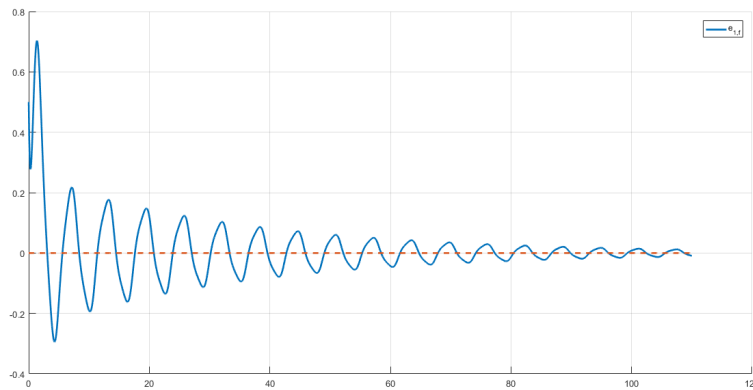
Figura 1.11: Erro de Identificação usando o Modelo por Regressão Linear para a planta \Sigma_p , com função de transferência G(s) = \frac{3}{s+1.5} , com parâmetros iniciais do Modelo \hat{a}_{1,f}(0) = 0.5 e \hat{k}_{1,f}(0) = 6 , com \lambda = 4 , para um passo de integração fixo de 10^{-3} segundos e 110 segundos de simulação
