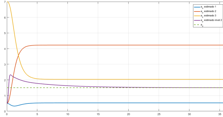
Figura 1.43: Estimativas do parâmetro a_p = 1.5 para a planta \Sigma_p para 3 Modelos por Regressão Linear e a estimativa de Segundo Nível Modificado entregue pela combinação convexa de coeficientes \alpha_{1,f} , \alpha_{2,f} e \alpha_{3,f} destas estimativas, com função de transferência G(s) = \frac{3}{s+1.5} , com parâmetros iniciais dos Modelos \hat{a}_{1,f}(0) = 0.5 e \hat{k}_{1,f}(0) = 1 , \hat{a}_{2,f}(0) = 0.5 e \hat{k}_{2,f}(0) = 11 , \hat{a}_{3,f}(0) = 7 e \hat{k}_{3,f}(0) = 1 , e valores iniciais dos coeficientes \alpha_{1,f}(0) = 0.5 , \alpha_{2,f}(0) = 0.5 e \alpha_{3,f}(0) = 0 , com \lambda = 4 e u(t) = 1 , para um passo de integração fixo de 10^{-3} segundos e 36 segundos de simulação
