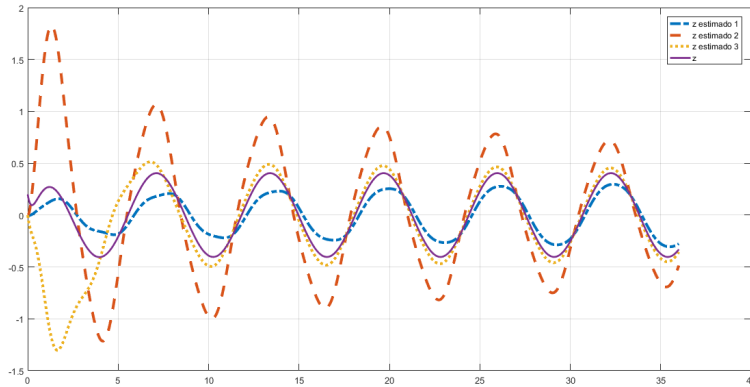
Figura 1.22: Saída da Planta e Estimativas da Saída da Planta usando 3 Modelos por Regressão Linear para a planta \Sigma_p , com função de transferência G(s) = \frac{3}{s+1.5} , com parâmetros iniciais do Modelos \hat{a}_{1,f}(0) = 0.5 e \hat{k}_{1,f}(0) = 1 , \hat{a}_{2,f}(0) = 0.5 e \hat{k}_{2,f}(0) = 11 , \hat{a}_{3,f}(0) = 7 e \hat{k}_{3,f}(0) = 1 , com \lambda = 4 , para um passo de integração fixo de 10^{-3} segundos e 36 segundos de simulação
