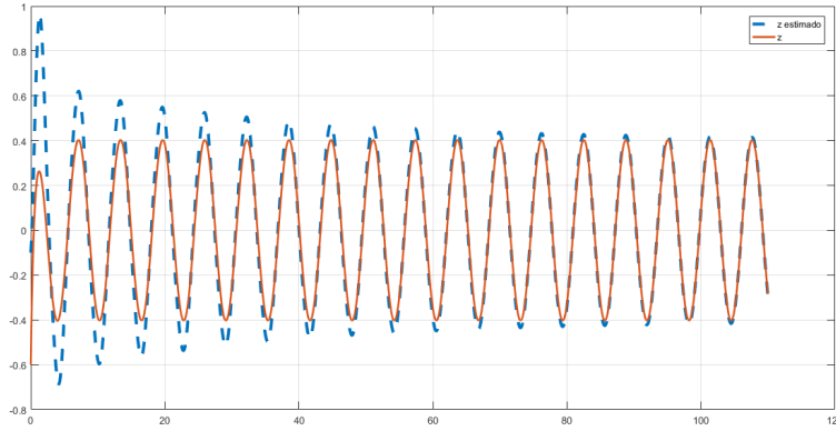
Figura 1.12: Saída da Planta Filtrada e Estimativa da Saída da Planta Filtrada usando o Modelo por Regressão Linear para a planta \Sigma_p , com função de transferência G(s) = \frac{3}{s+1.5} , com parâmetros iniciais do Modelo \hat{a}_{1,f}(0) = 0.5 e \hat{k}_{1,f}(0) = 6 , com \lambda = 4 , para um passo de integração fixo de 10^{-3} segundos e 110 segundos de simulação
