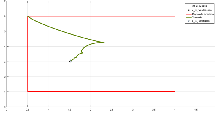
Figura 1.35: Trajetória dos parâmetros \hat{a}_{n2,f} e \hat{k}_{n2,f} da Adaptação de Segundo Nível no espaço de parâmetros usando 8 Modelos por Regressão Linear para a planta \Sigma_p , com função de transferência G(s) = \frac{3}{s+1.5} , com parâmetros iniciais dos Modelos \hat{a}_{1,f}(0) = 0.5 e \hat{a}_{1,f}(0) = 0.5 e \hat{k}_{1,f}(0) = 1 , \hat{a}_{2,f}(0) = 2.25 e \hat{k}_{2,f}(0) = 1 , \hat{a}_{3,f}(0) = 4 e \hat{k}_{3,f}(0) = 1 , \hat{a}_{3,f}(0) = 4 e \hat{k}_{3,f}(0) = 1 , \hat{a}_{4,f}(0) = 4 e \hat{k}_{4,f}(0) = 3.5 , \hat{a}_{5,f}(0) = 4 e \hat{k}_{5,f}(0) = 6 , \hat{a}_{6,f}(0) = 2.25 e \hat{k}_{6,f}(0) = 6 , \hat{a}_{7,f}(0) = 0.5 e \hat{k}_{7,f}(0) = 6 , \hat{a}_{8,f}(0) = 0.5 e \hat{k}_{8,f}(0) = 3.5 , e valor inicial de \alpha_{7,sp}(0) = 1 , com os demais coeficientes iguais a zero inicialmente, com \lambda = 4 , para um passo de integração fixo de 10^{-3} segundos e 20 segundos de simulação
