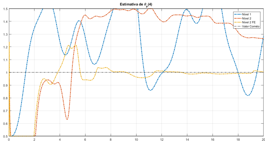
Figura 5.4: Comportamento das estimativas do coeficiente b_2 do polinômio N_p(s) para o Modelo de Primeiro Nível, Adaptação de Segundo Nível sem Fator de Esquecimento e Adaptação de Segundo Nível com Fator de Esquecimento.
