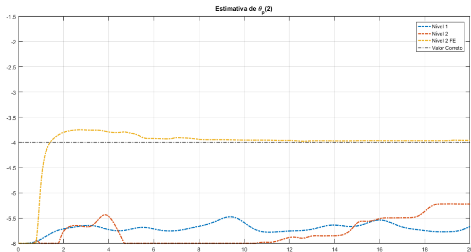
Figura 5.2: Comportamento das estimativas do coeficiente a_2 do polinômio D_p(s) para o Modelo de Primeiro Nível, Adaptação de Segundo Nível sem Fator de Esquecimento e Adaptação de Segundo Nível com Fator de Esquecimento.
