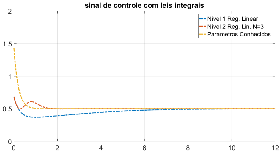
Figura 3.5: Sinal de controle para Controle Adaptativo Indireto baseado Modelo de Identificação por Regressão Linear, Controle Adaptativo Indireto baseado em Adaptação de Segundo Nível com N=3 e Controle com Parâmetros Conhecidos da Planta de Ordem 1, 12 segundos de simulação
