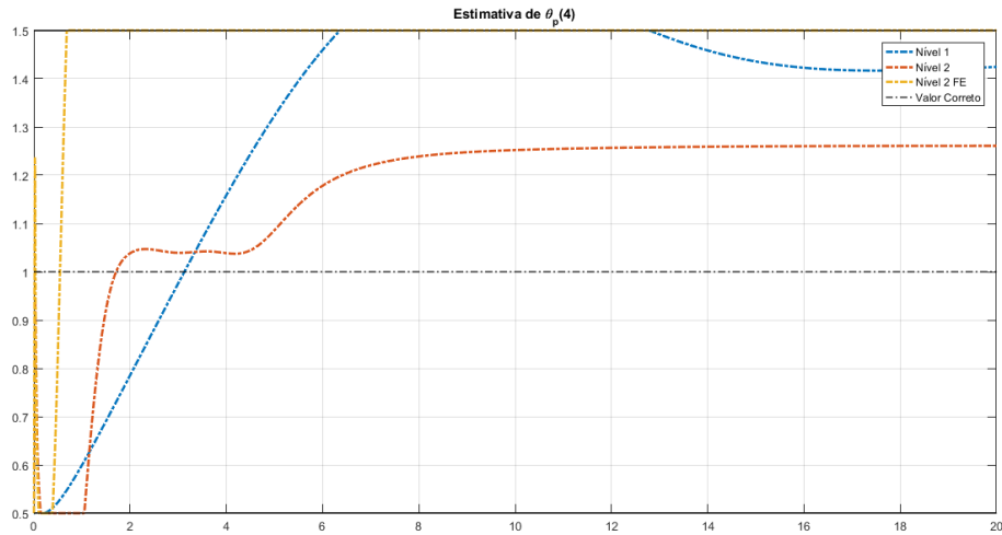
Figura 5.12: Comportamento das estimativas do coeficiente b_2 do polinômio N_p(s) para o Modelo de Primeiro Nível, Adaptação de Segundo Nível sem Fator de Esquecimento e Adaptação de Segundo Nível com Fator de Esquecimento com referência degrau.
