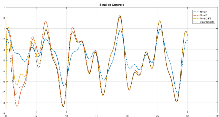
Figura 5.6: Sinal de Controle gerado pelo controlador com base nas estimativas do Modelo de Primeiro Nível, Adaptação de Segundo Nível sem Fator de Esquecimento e Adaptação de Segundo Nível com Fator de Esquecimento.
