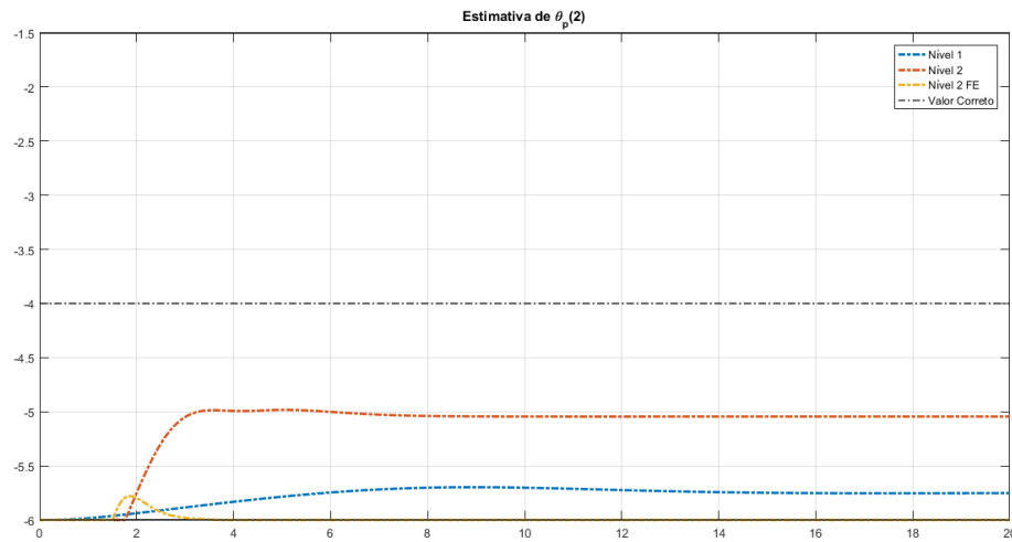
Figura 5.10: Comportamento das estimativas do coeficiente a_2 do polinômio D_p(s) para o Modelo de Primeiro Nível, Adaptação de Segundo Nível sem Fator de Esquecimento e Adaptação de Segundo Nível com Fator de Esquecimento com referência degrau.
