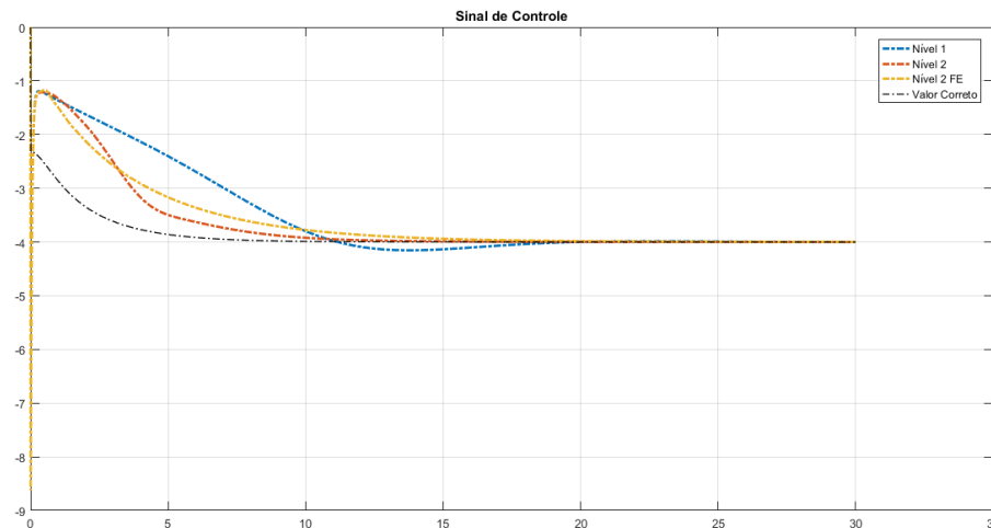
Figura 5.14: Sinal de Controle gerado pelo controlador com base nas estimativas do Modelo de Primeiro Nível, Adaptação de Segundo Nível sem Fator de Esquecimento e Adaptação de Segundo Nível com Fator de Esquecimento com referência degrau.
