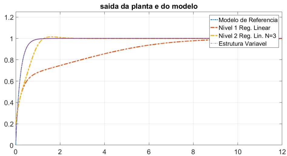
Figura 3.3: Saída da planta \Sigma_p de ordem 1 para o Controle Adaptativo Indireto baseado Modelo de Identificação por Regressão Linear, Controle Adaptativo Indireto baseado em Adaptação de Segundo Nível com N=3 , Controle com Estrutura Variável e Controle com Parâmetros Conhecidos, 12 segundos de simulação
