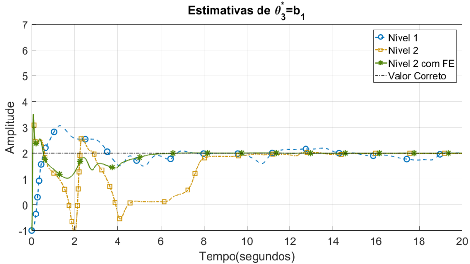
Figura 4.3: Comportamento das estimativas do coeficiente b_1 do polinômio N_p(s) para o modelo de primeiro nível, SLA e SLAFF.
