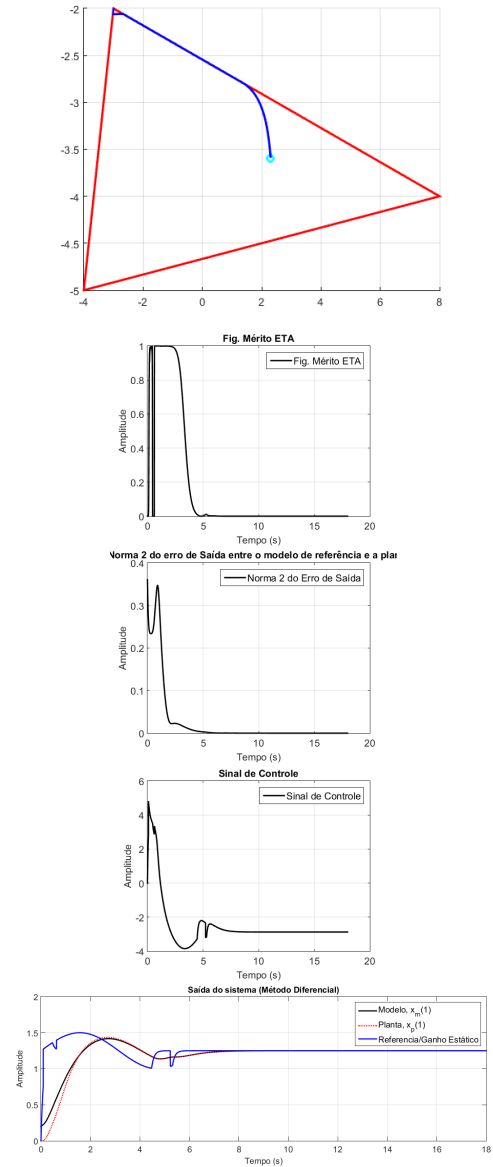
Figura 1: a)Trajetória dos parâmetros b)Comportamento da figura de Mérito \eta c)Norma do vetor de erros entre as variáveis de estado da planta e do modelo de referência d)Sinal de Controle e)Comportamento da Saída da Planta, Referência/Ganho Estático e Saída do Modelo de Referência
