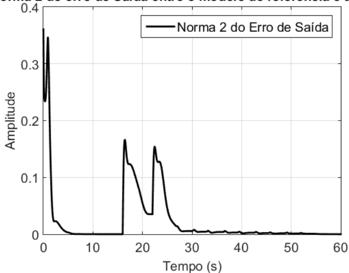
Figura: Norma do vetor de erros de saída
