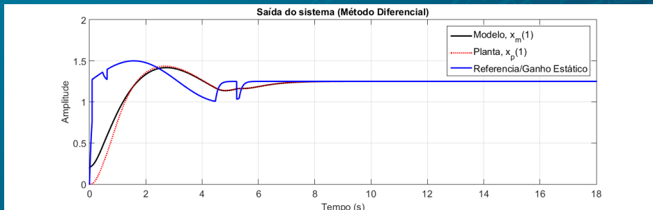
Figura: Comportamento da Saída da Planta, Referência/Ganho Estático e Saída do Modelo de Referência
