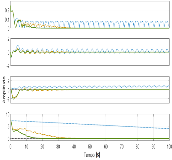
Figura 1: a) norma 2 do erro de saída e_o(t) , b) erro de controle dado por e_u(t) = u^*(t) - u(t) , c) erro paramétrico dado por \phi_1(t) = \hat{a}_1 - a_1 , d) erro paramétrico dado por \phi_2(t) = \hat{a}_2 - a_2 . As linhas pontilhadas azuis correspondem à equação (7), as linhas tracejadas amarelas à (23), e as linhas cheias verdes à (33).
