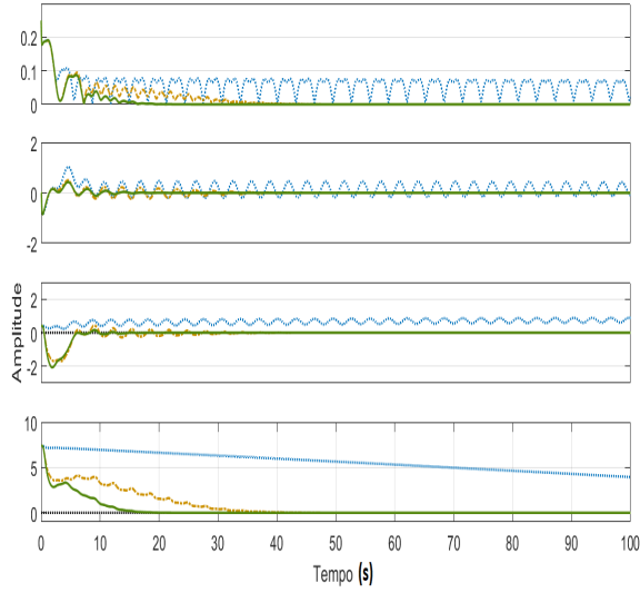
Figura 1: a) norma 2 do erro de saída e_o(t) , b) erro de controle dado por e_u(t) = u^*(t) - u(t) , c) erro paramétrico dado por \phi_1(t) = \hat{a}_1 - a_1 , d) erro paramétrico dado por \phi_2(t) = \hat{a}_2 - a_2 . As linhas pontilhadas azuis correspondem à equação (7), as linhas tracejadas amarelas à (23), e as linhas cheias verdes à (33).
