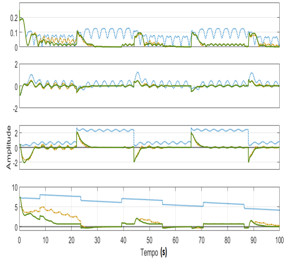
Figura 3: a) norma 2 do erro de saída e_o(t) , b) erro de controle dado por e_u(t) = u^*(t) - u(t) , c) erro paramétrico dado por \phi_1(t) = \hat{a}_1 - a_1 , d) erro paramétrico dado por \phi_2(t) = \hat{a}_2 - a_2 . As linhas pontilhadas azuis correspondem à equação (7), as linhas tracejadas amarelas à (23), e as linhas cheias verdes à (33).
