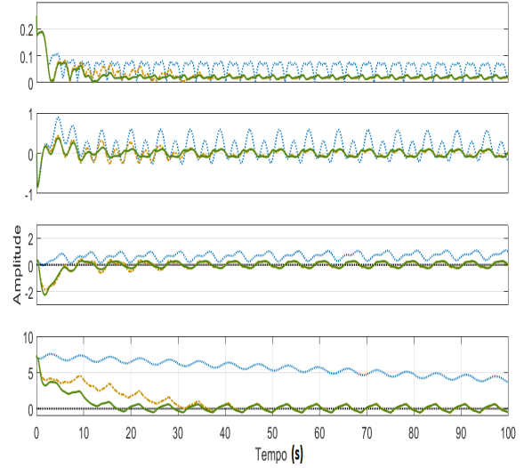
Figura 2: a) norma 2 do erro de saída e_o(t) , b) erro de controle dado por e_u(t) = u^*(t) - u(t) , c) erro paramétrico dado por \phi_1(t) = \hat{a}_1 - a_1 , d) erro paramétrico dado por \phi_2(t) = \hat{a}_2 - a_2 . As linhas pontilhadas azuis correspondem à equação (7), as linhas tracejadas amarelas à (23), e as linhas cheias verdes à (33).
