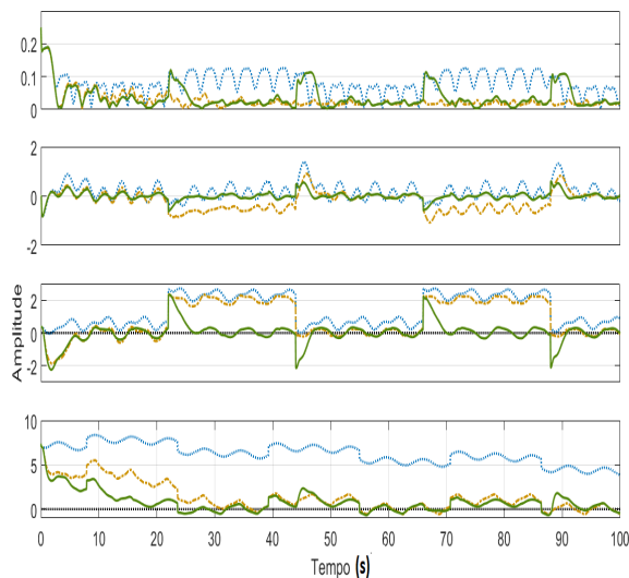
Figura 4: a) norma 2 do erro de saída e_o(t) , b) erro de controle dado por e_u(t) = u^*(t) - u(t) , c) erro paramétrico dado por \phi_1(t) = \hat{a}_1 - a_1 , d) erro paramétrico dado por \phi_2(t) = \hat{a}_2 - a_2 . As linhas pontilhadas azuis correspondem à equação (7), as linhas tracejadas amarelas à (23), e as linhas cheias verdes à (33).
