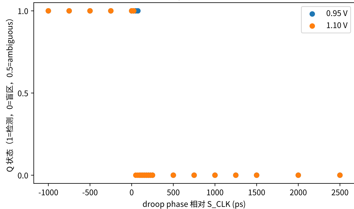
图 T0-2：单 probe 相位敏感窗口
