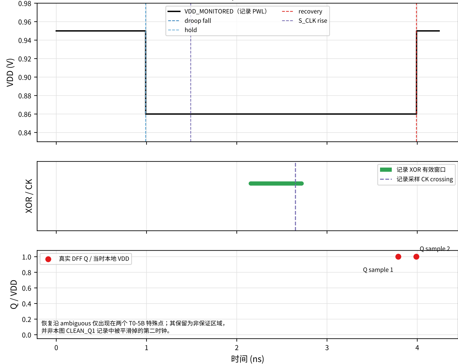
图 T0-1 : 0.95 V / L2 / 3002 ps 长脉冲的记录事件与真实 Q 采样
