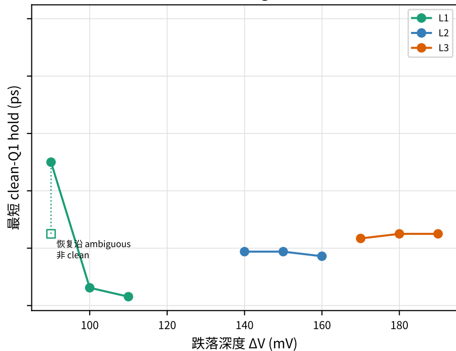
1.10 V：margin 比较
