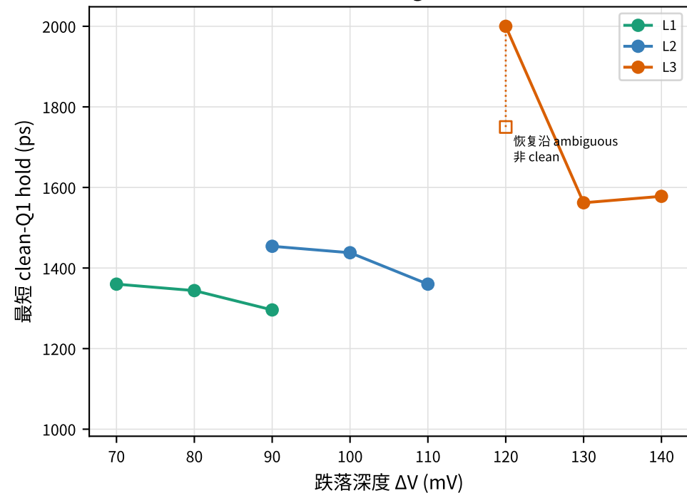
0.95 V：margin 比较
