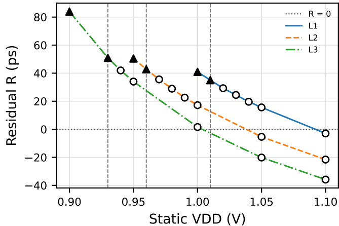
1.10 V baseline
