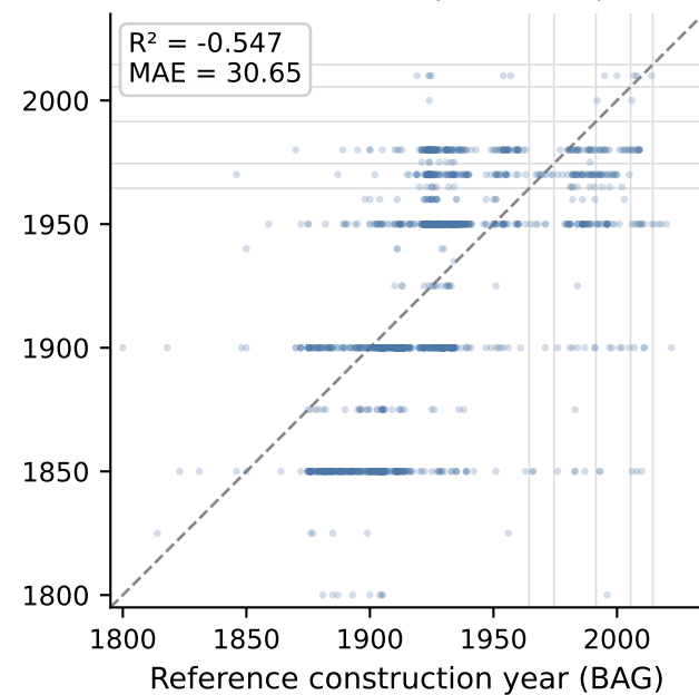
InternVL3-2B (zero-shot)
