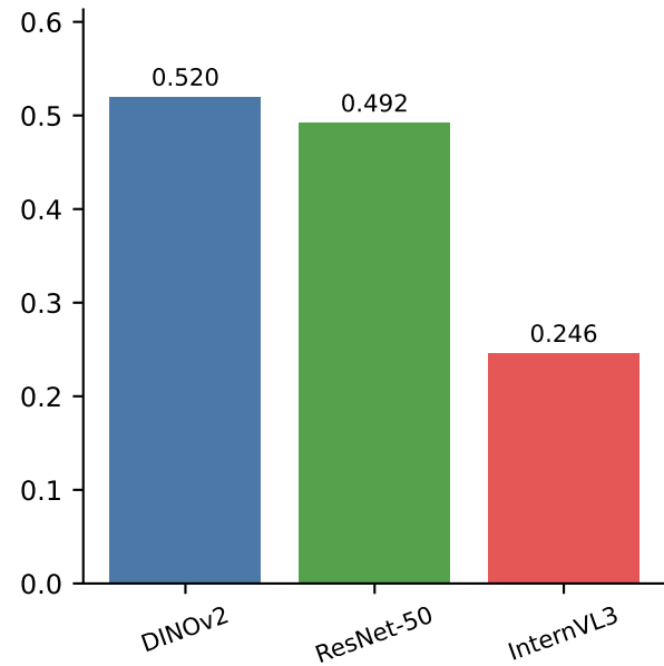
type macro-F1
