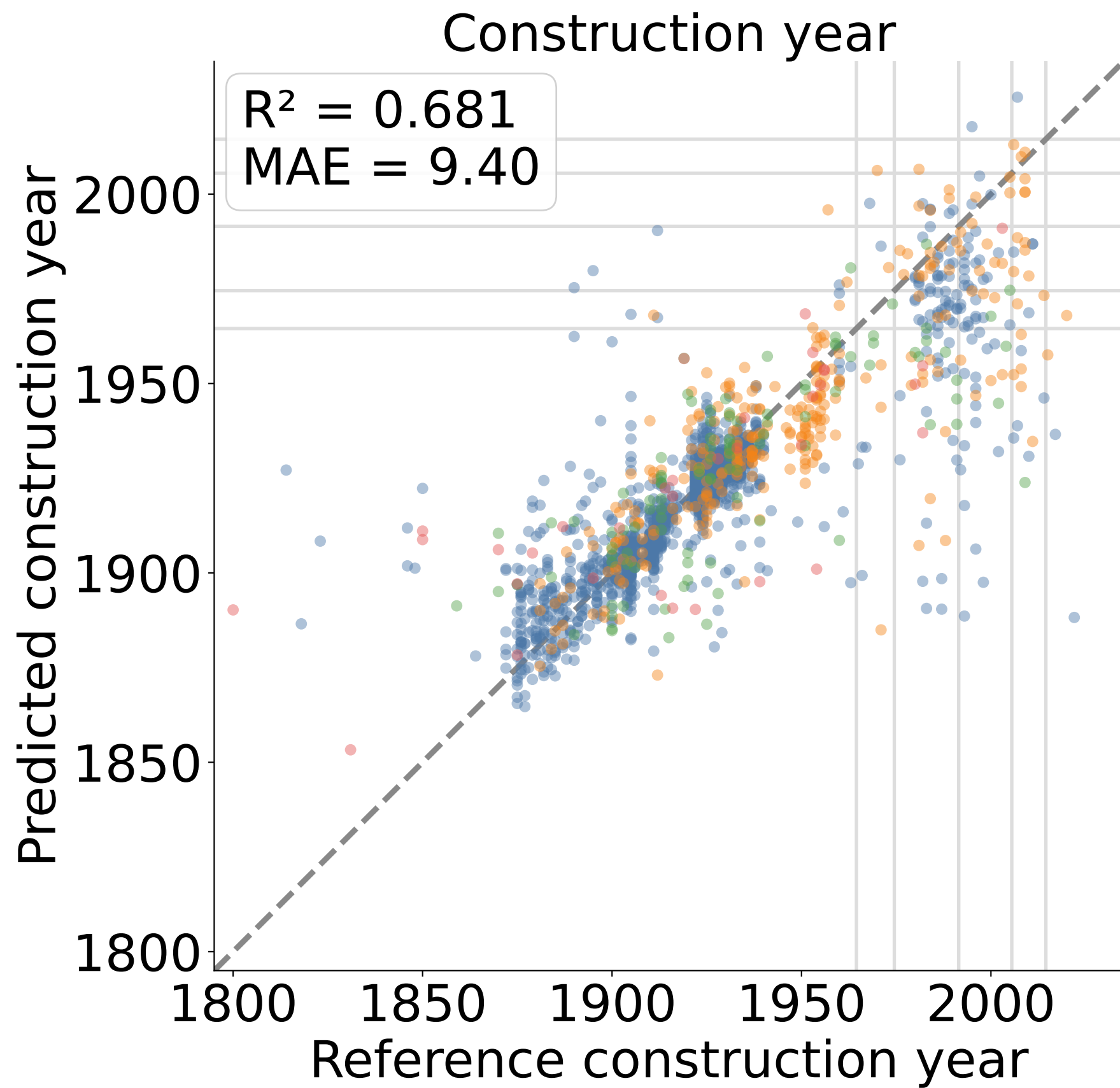
DINOv2
