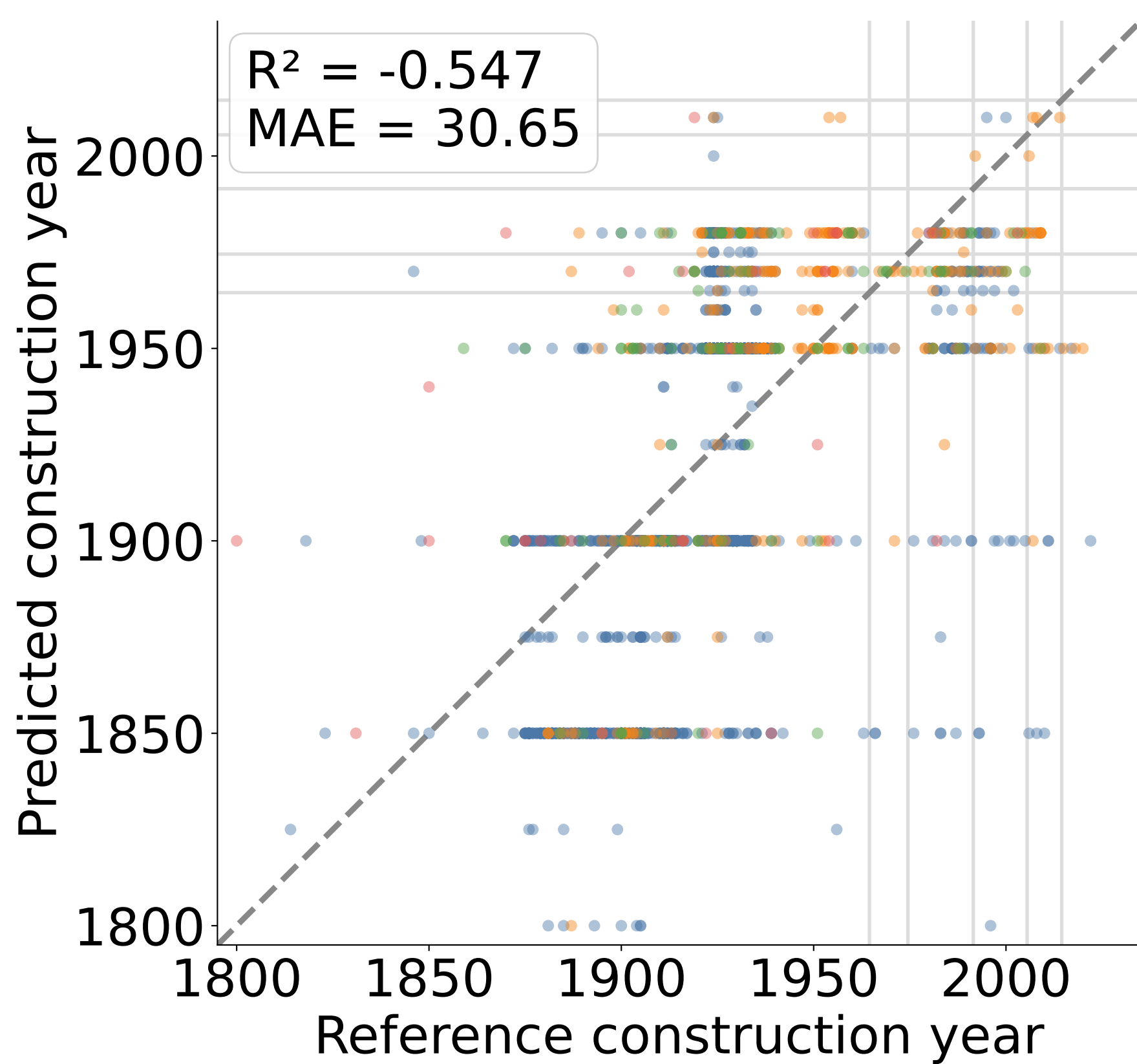
InternVL3-2B
