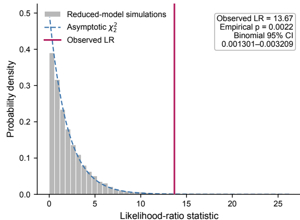
(a) NGRIP-MIS6
