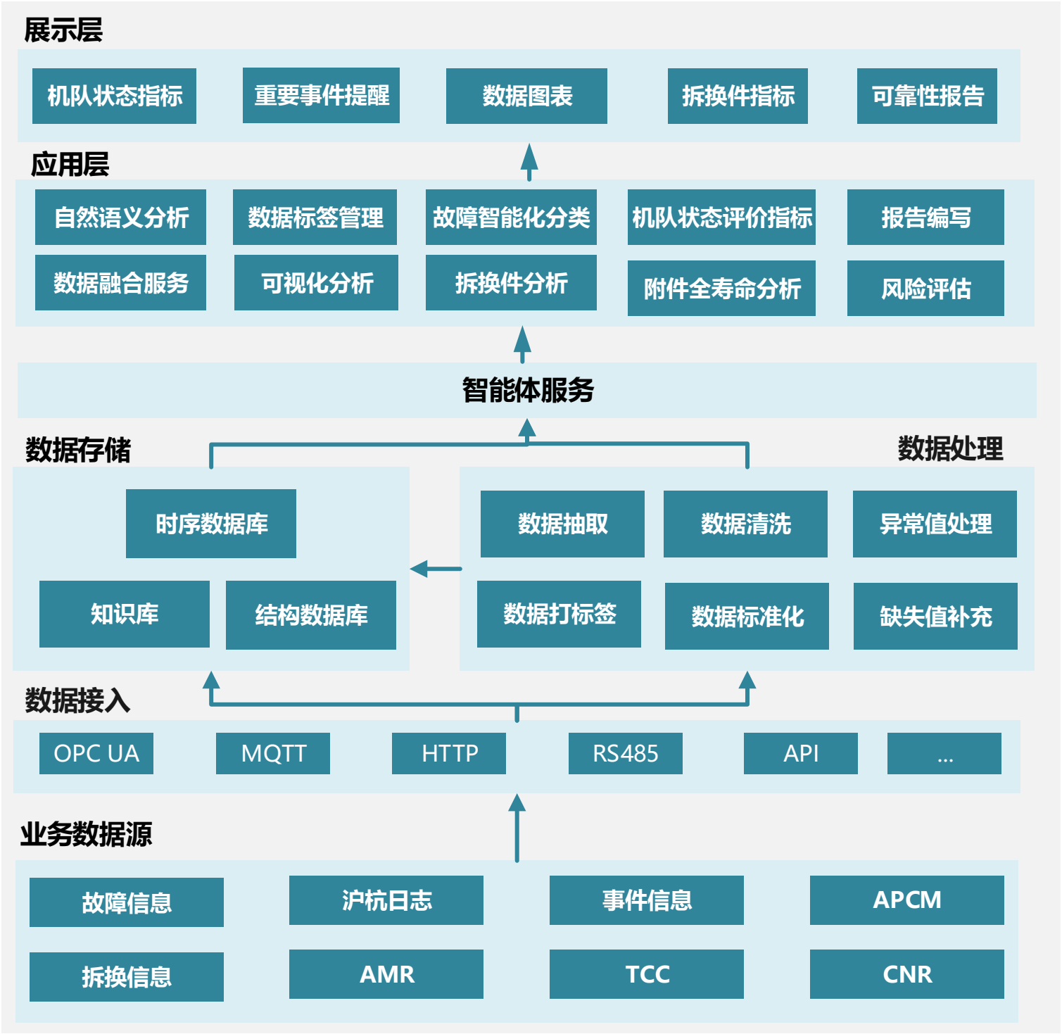
Ameco可靠性分析功能架构图
