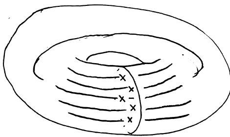
Kuva 12: Torus koostuu erillisistä ympyröistä: \mathbb{T}^2 = \bigsqcup_{p \in \mathbb{D}^2} \{p\} \times \mathbb{S}^1 .
