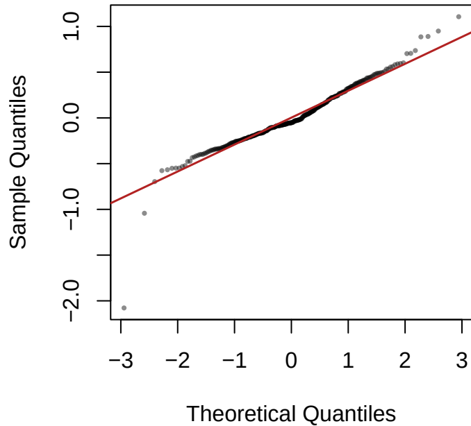
Normal Q-Q
